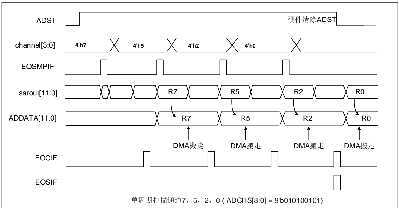
图 13-6 单周期扫描下使能通道转换时序图（通道方向从低到高）
