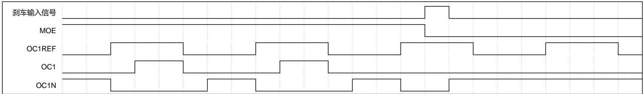
图 19-11 响应刹车的输出 (OISx=0, OISxN=1)
