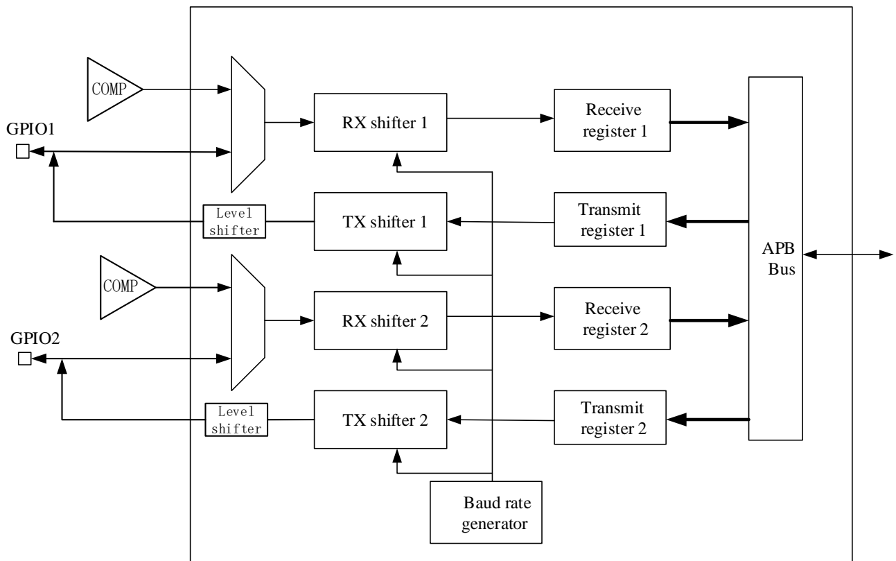
图 26-1 CSM 功能框图
