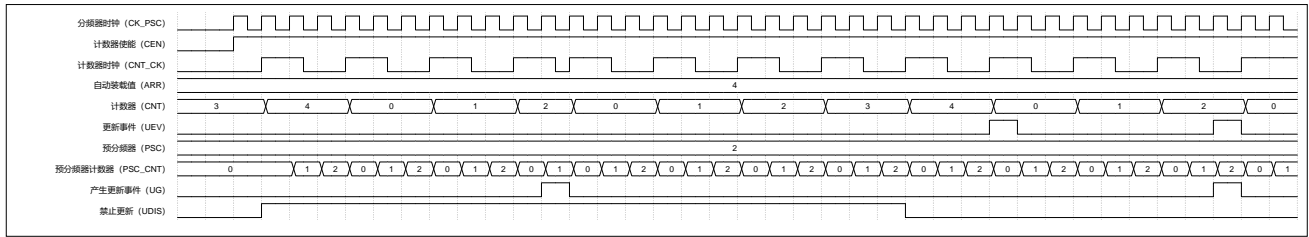
图 16-7 递增计数模式 (UDIS=1 禁止产生更新事件)
