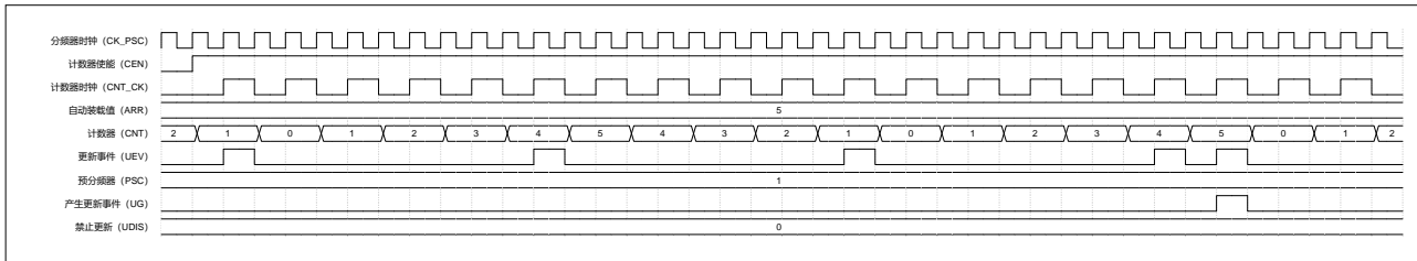
图 16-10 中央计数模式（UDIS=0）
