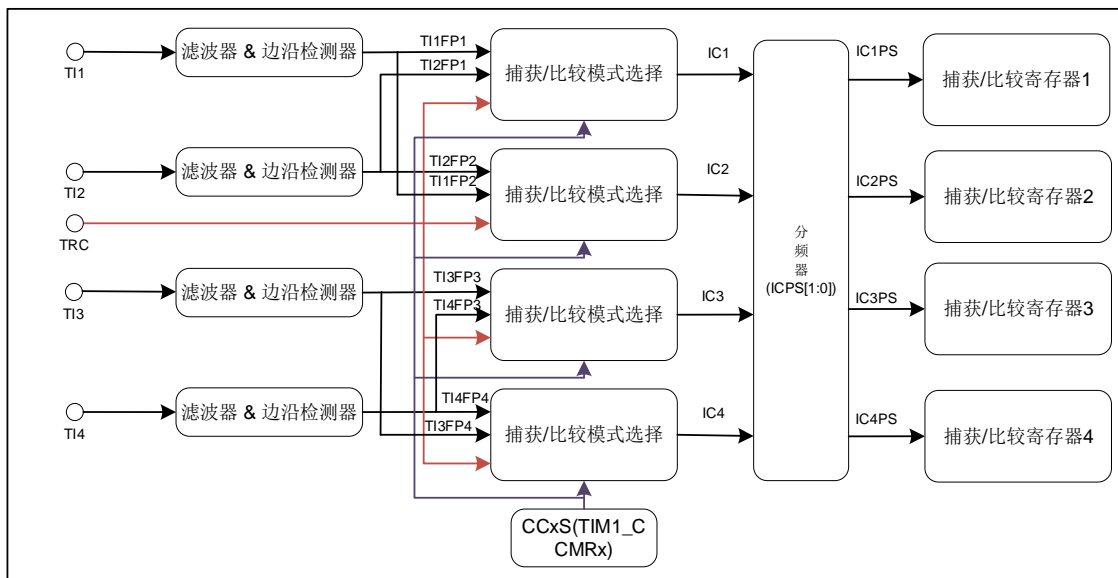
图 15-15 TIMx 输入捕获结构图
