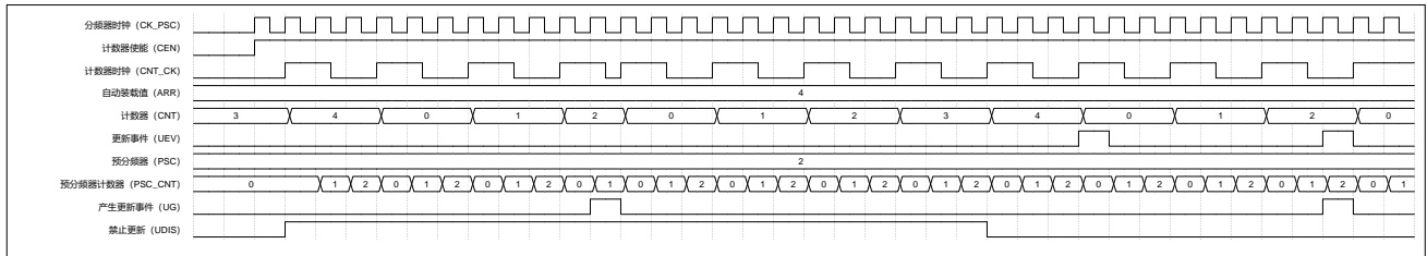
图 17-7 递增计数模式 (UDIS=1 禁止产生更新事件)
