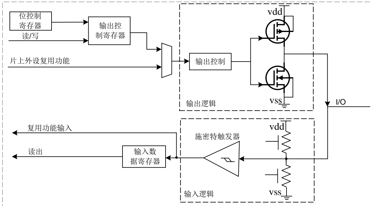
图 9-4 复用功能配置
