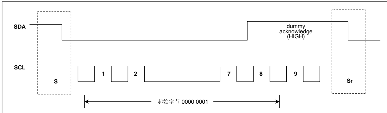
图 25-8 起始字节传输
