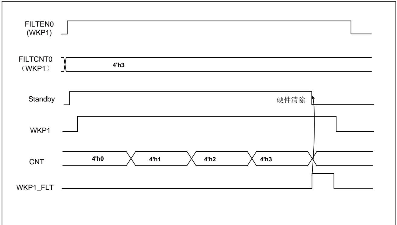
图 3-4 Standby 模式唤醒滤波功能波形图
