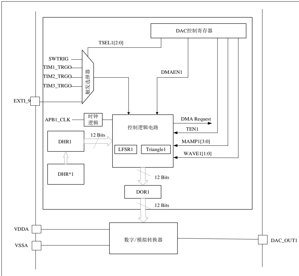
图 14-1 DAC 单通道功能框图
