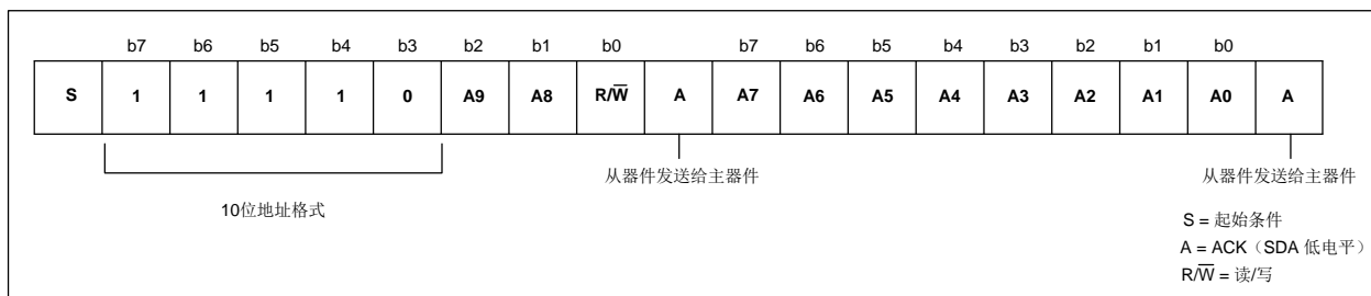
图 25-4 10 位地址格式
