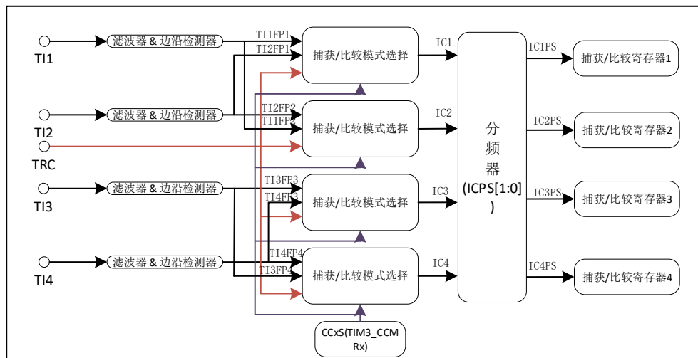
图 17-12 TIM3 输入捕获结构图
