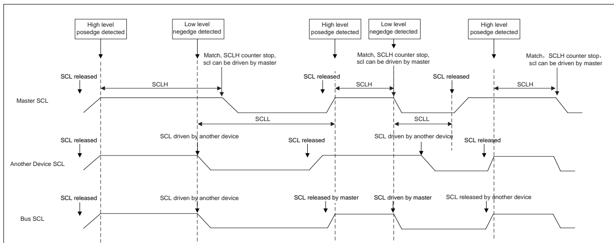
图 25-16 时钟同步（时序图）
