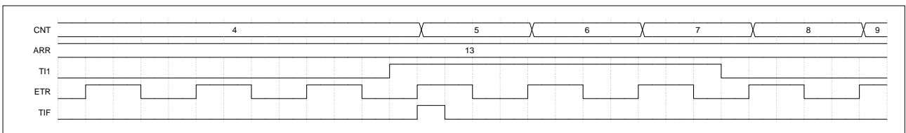
图 15-36 外部时钟模式 2+从模式（触发模式）控制时序图
