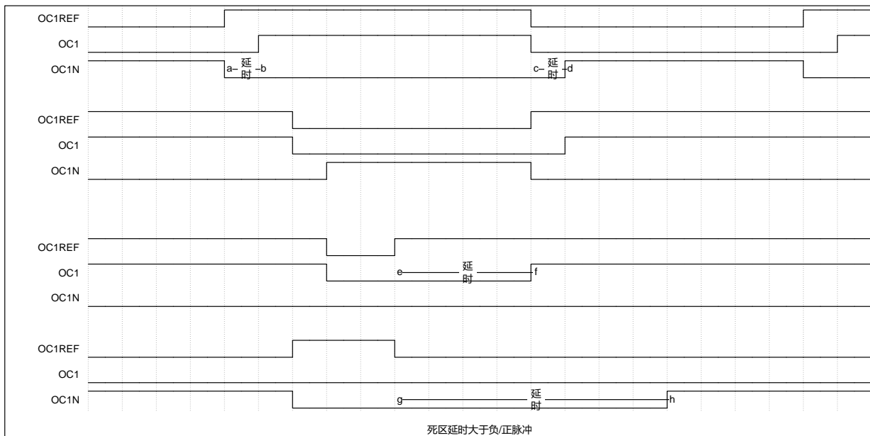
图 19-9 死区插入
