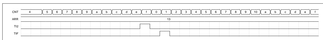
图 15-33 复位模式的控制时序图
