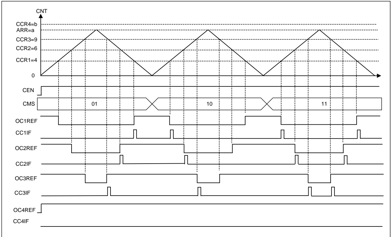
图 16-18 中央对齐 PWM 模式 1 的波形
