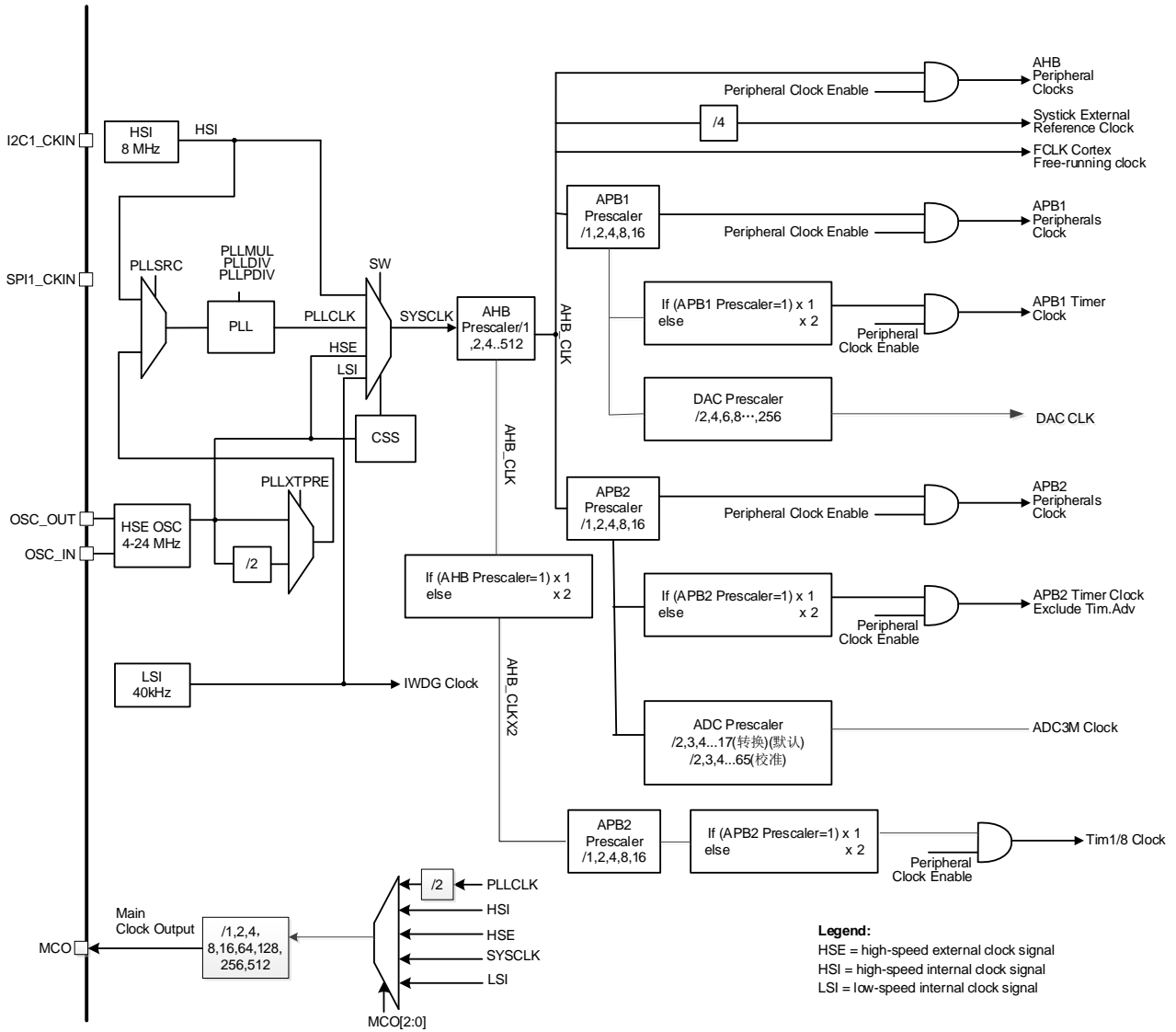
图 5-2 时钟树
