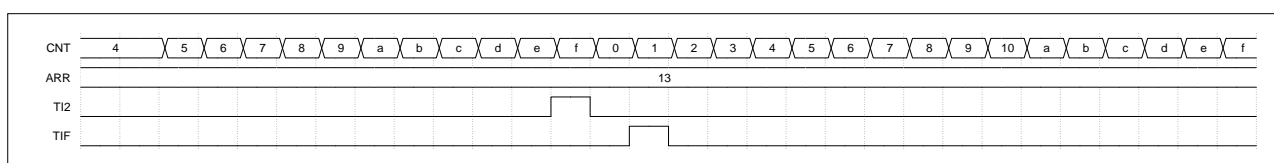
图 16-23 复位模式的控制时序图
