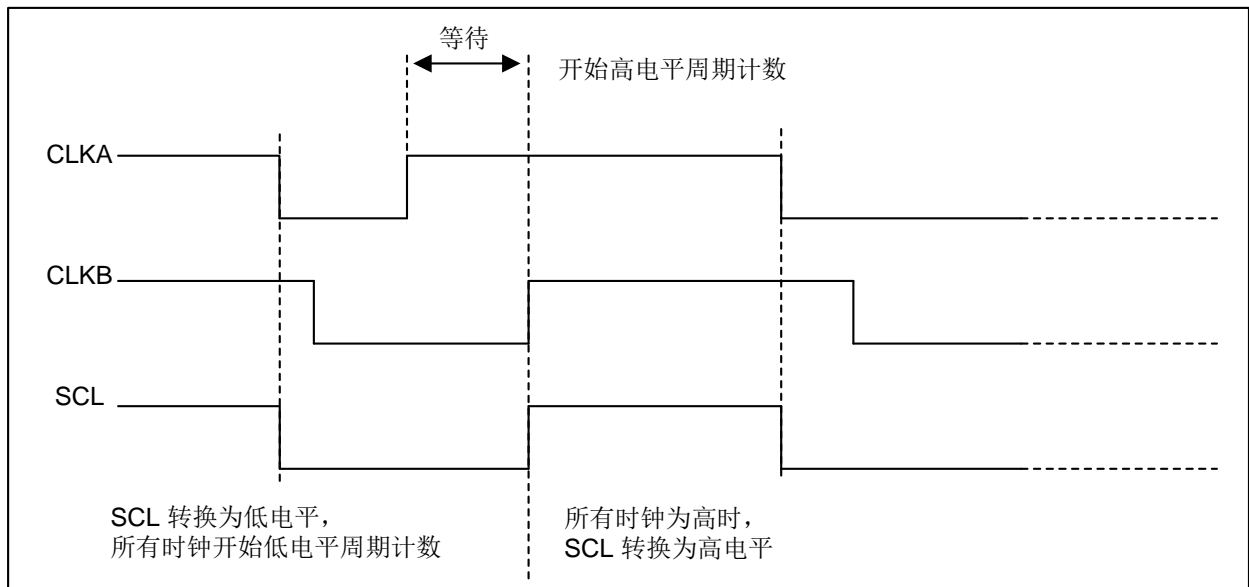
图 25-15 时钟同步（示意图）
