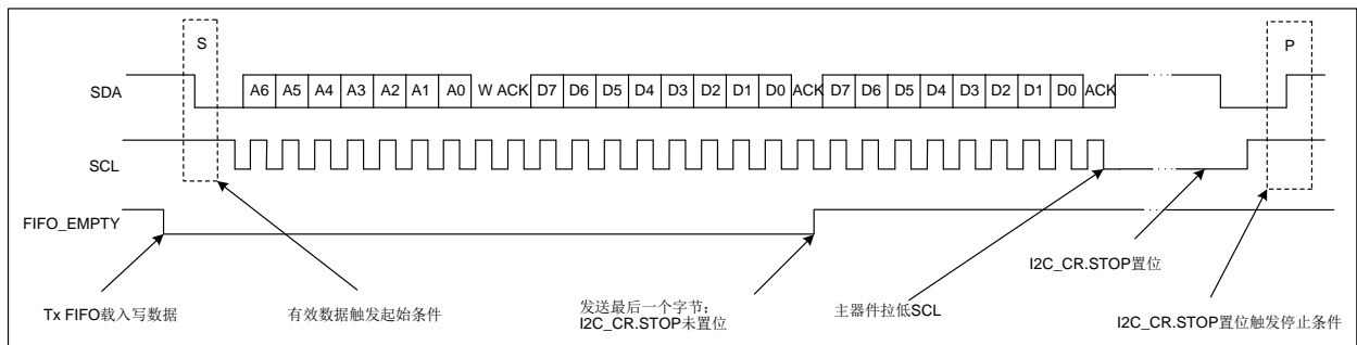
图 25-10 主发送，TX FIFO 为空
