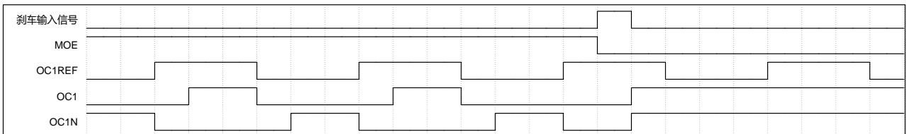
图 19-13 响应刹车的输出 (OISx=1, OISxN=1)
