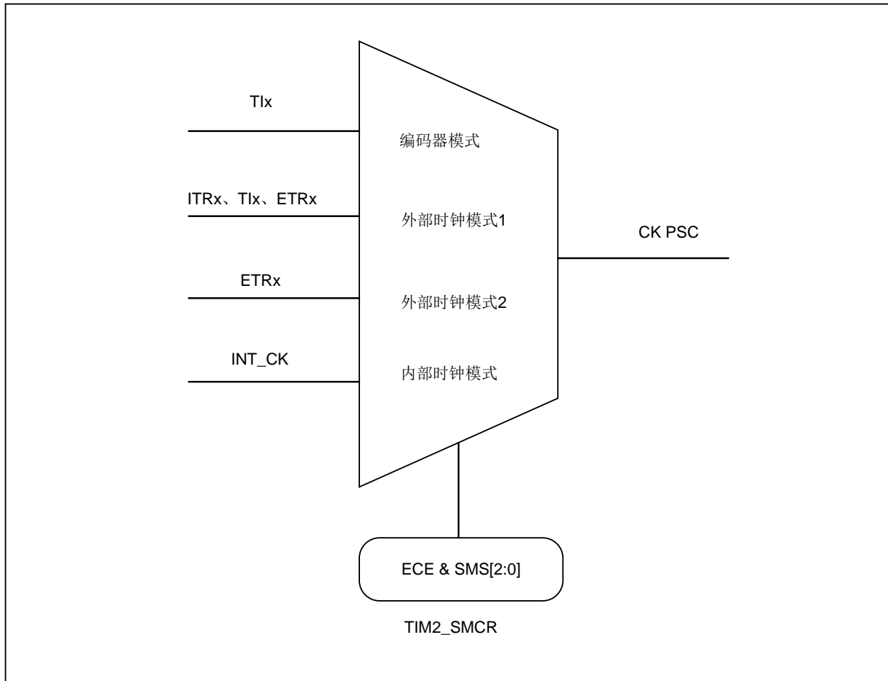
图 16-2 时钟选择
