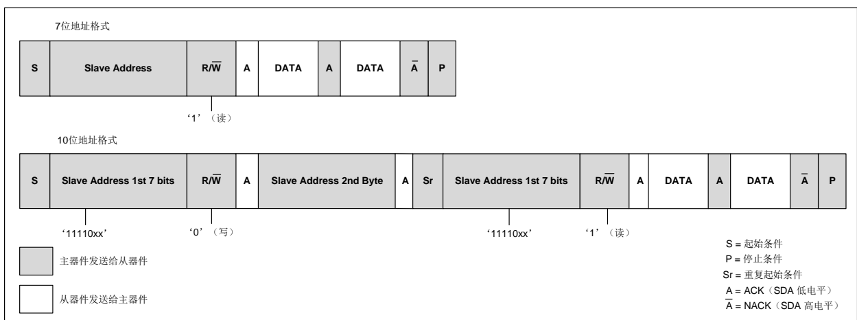
图 25-6 主接收协议
