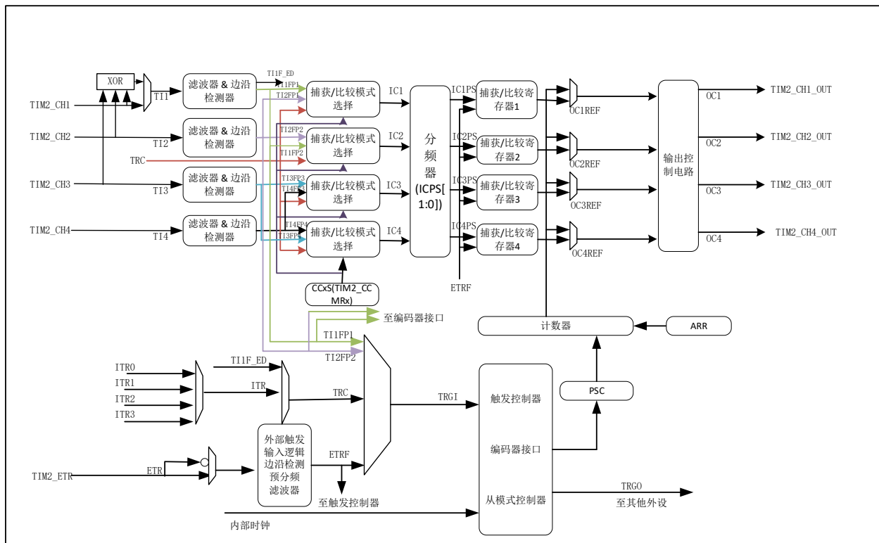
图 16-1 TIM2 结构图
