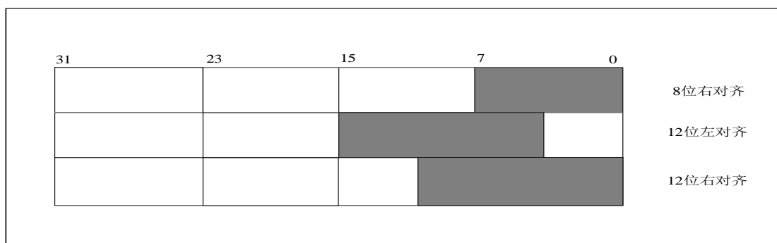
图 14-2 DAC 的数据保持寄存器的不同数据格式
