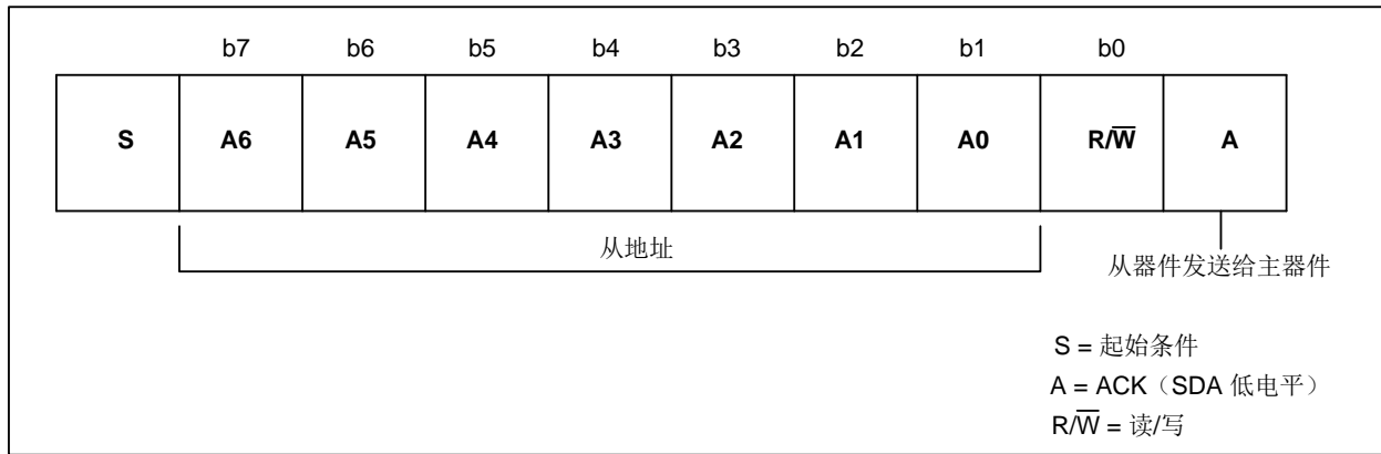
图 25-3 7 位地址格式
