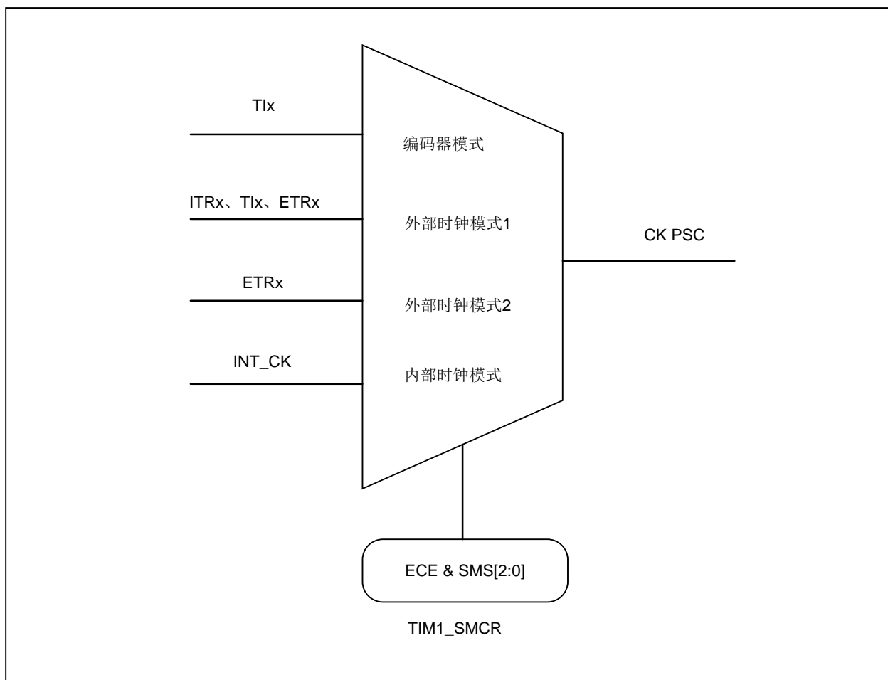
图 15-2 时钟选择
