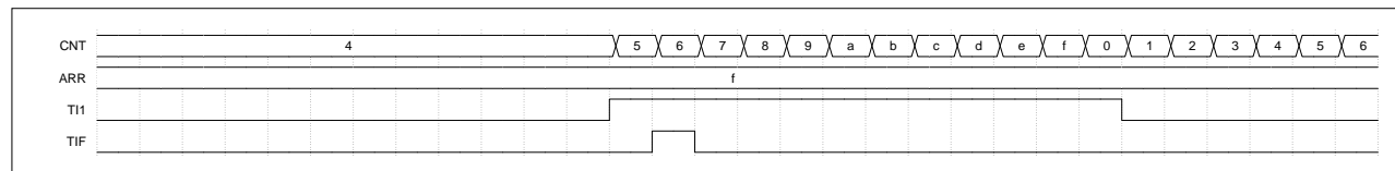
图 16-25 触发器模式下的控制时序图
