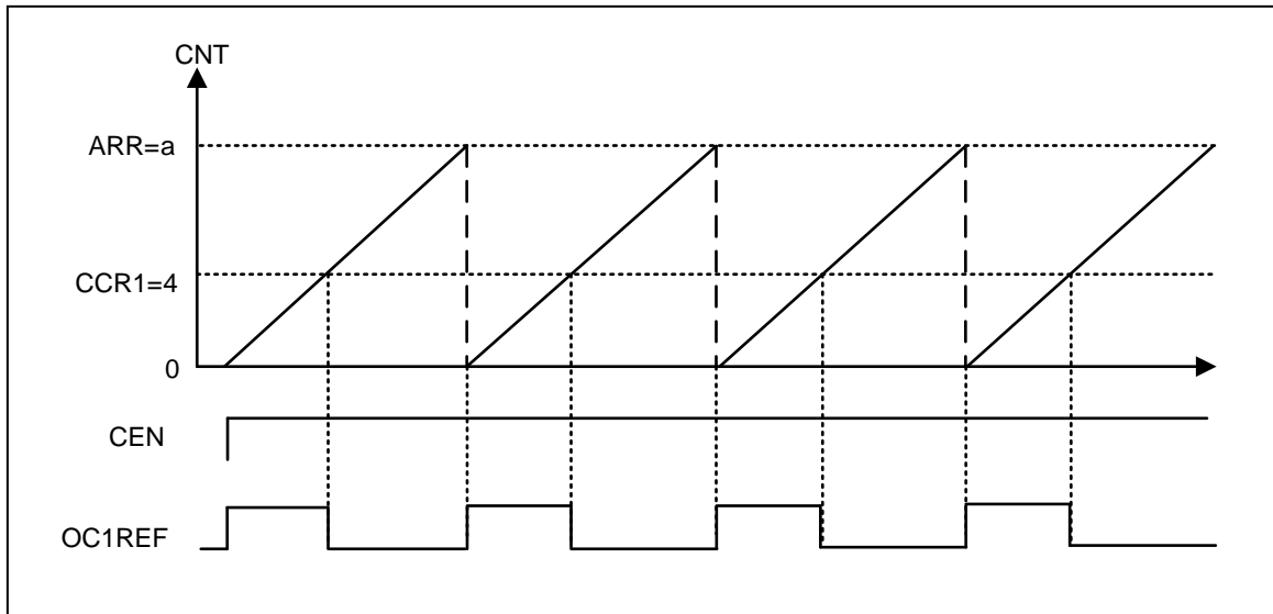
图 18-8 边沿对齐递增计数时 PWM 模式 1 的波形
