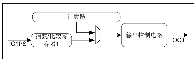
图 18-6 比较输出部分结构图
