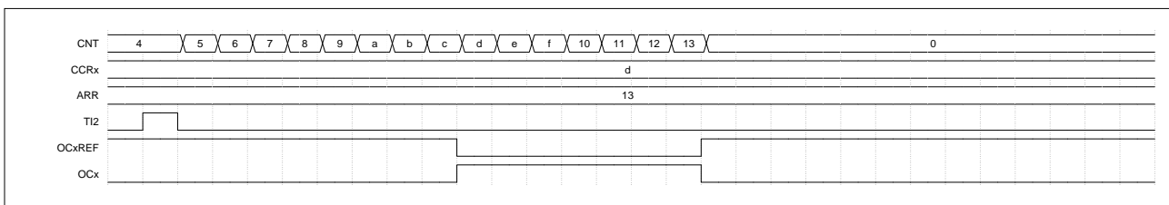
图 17-20 单脉冲模式
