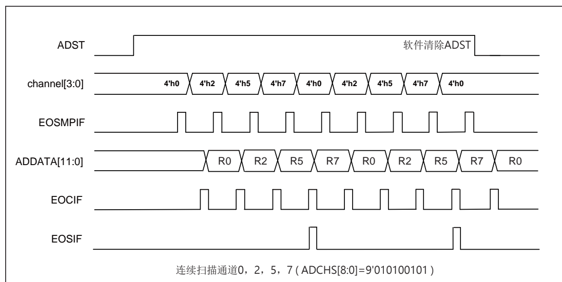
图 13-8 连续扫描模式使能通道转换时序图 (通道方向由低到高)
