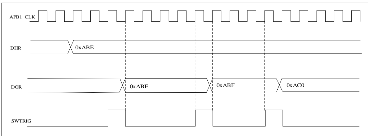
图 14-4 带三角波生成的 DAC 转换（使能软件触发）
