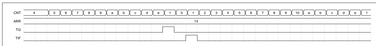
图 17-23 复位模式的控制时序图
