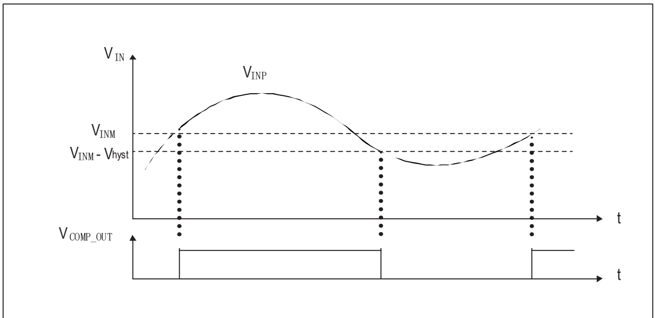
图 12-2 比较器的迟滞
