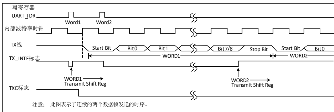
图 23-4 发送时状态位变化
