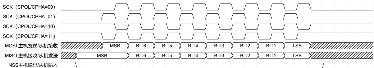
图 24-3 数据时钟时序图
