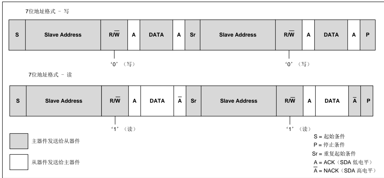
图 25-7 带 RESTART (SR) 信号的主发送和接收协议
