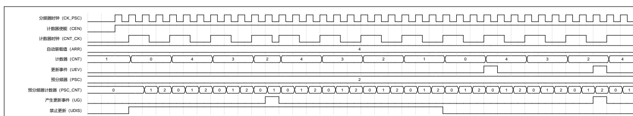
图 15-11 中央计数模式（UDIS=1 禁止产生更新事件）
