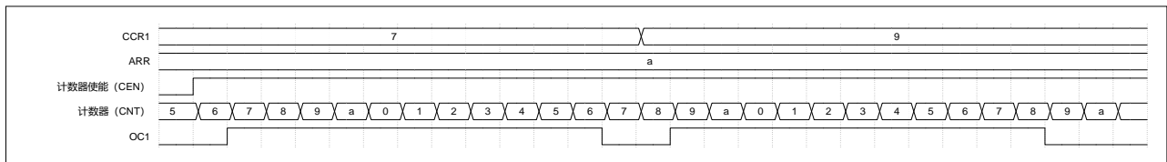
图 15-18 比较输出模式，OC1 信号在匹配时翻转
