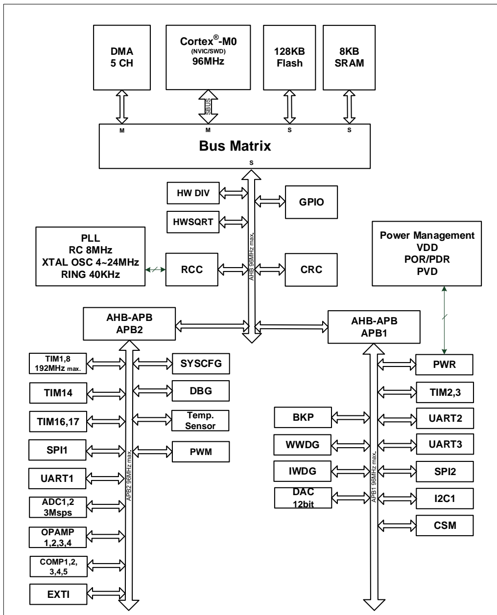
图 1-1 系统架构框图
