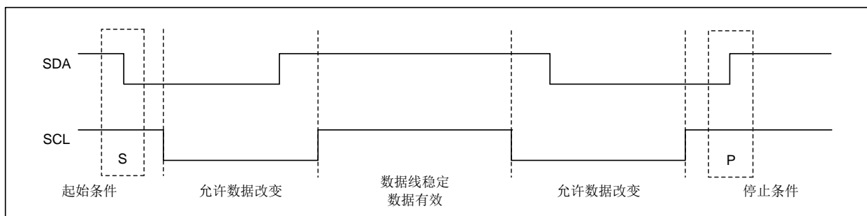
图 25-2 起始和停止条件
