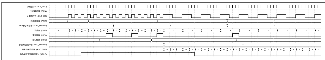
图 19-2 自动预装载
