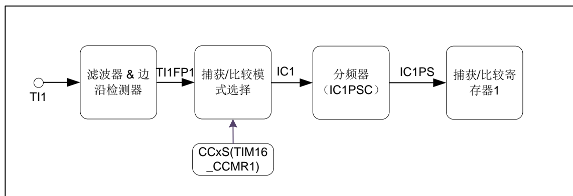
图 19-5 TIMx 输入捕获结构图
