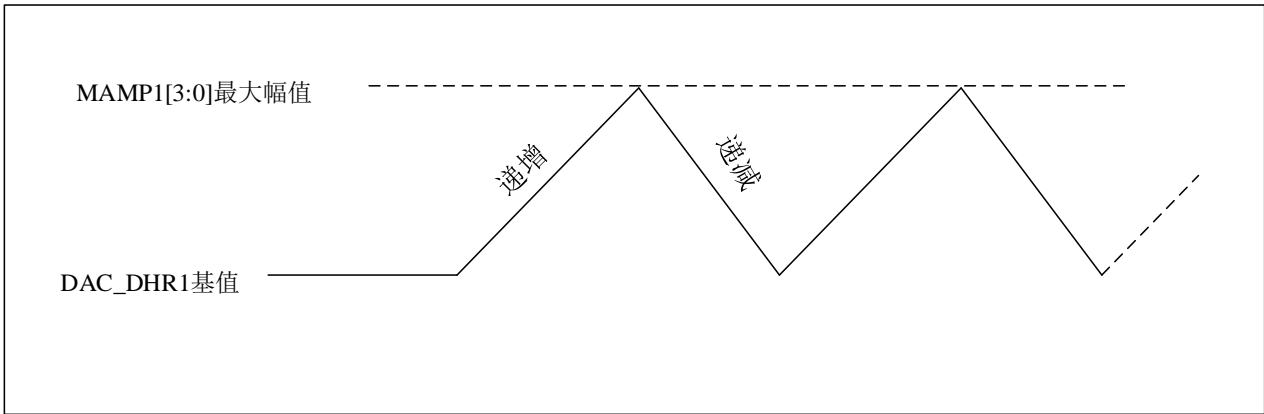
图 14-3 DAC 三角波生成
