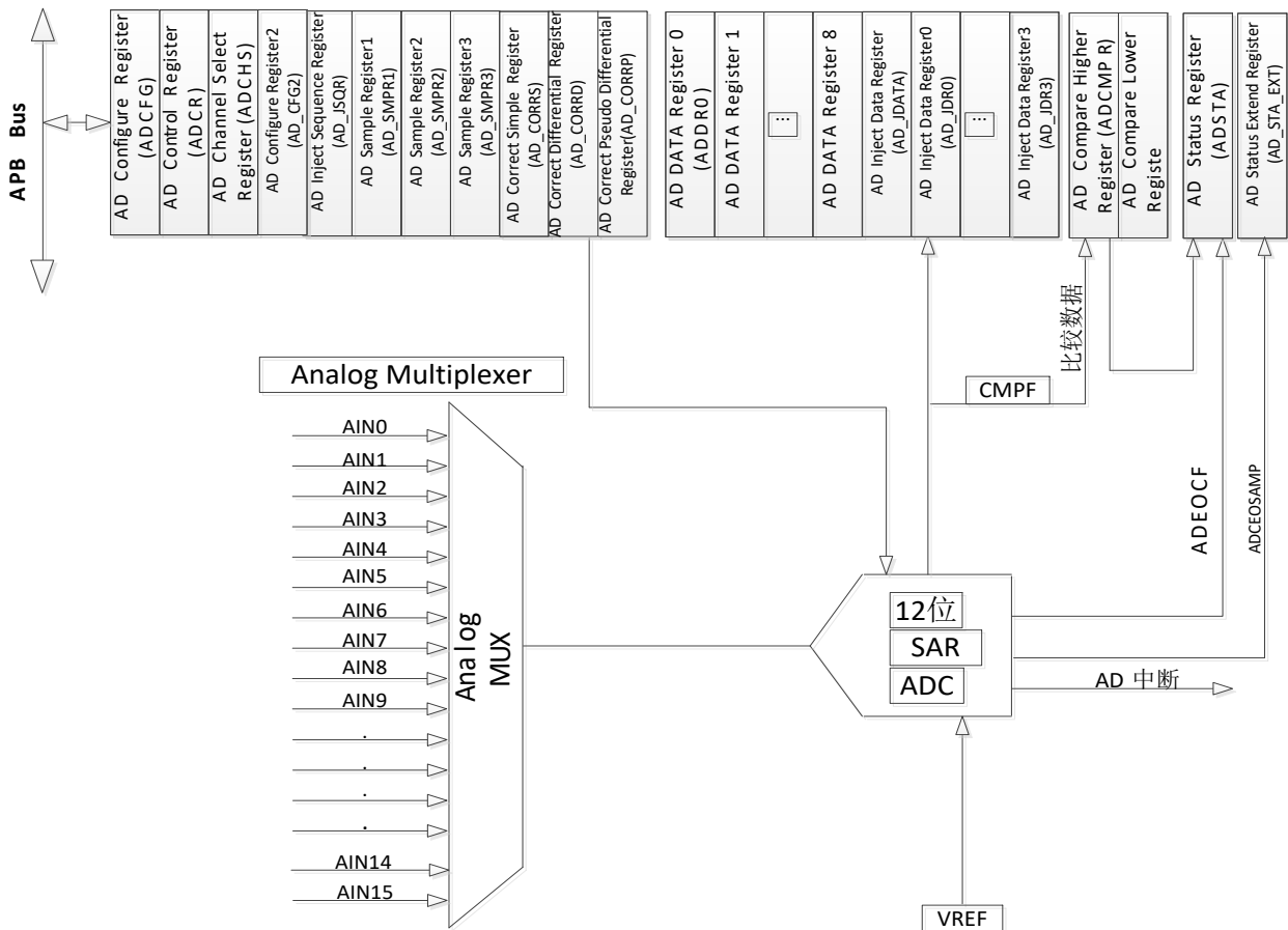
图 13-1 ADC 系统框图
