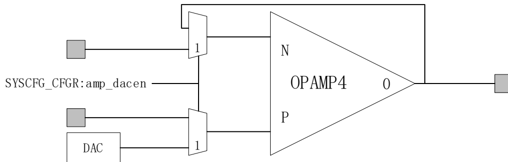
图 27-1 OPAMP4 功能框图
