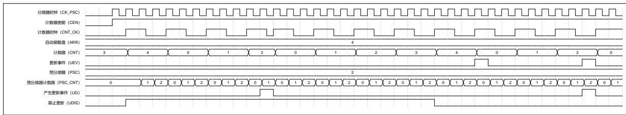
图 18-4 递增计数模式 (UDIS=1 禁止产生更新事件)
