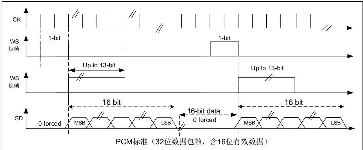
图 24-7 PCM 标准示意图
