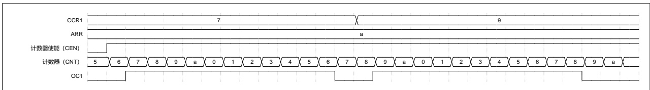
图 17-15 比较输出模式，OC1 信号在匹配时翻转
