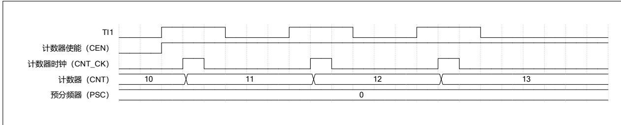
图 16-3 外部时钟模式 1 下的控制电路
