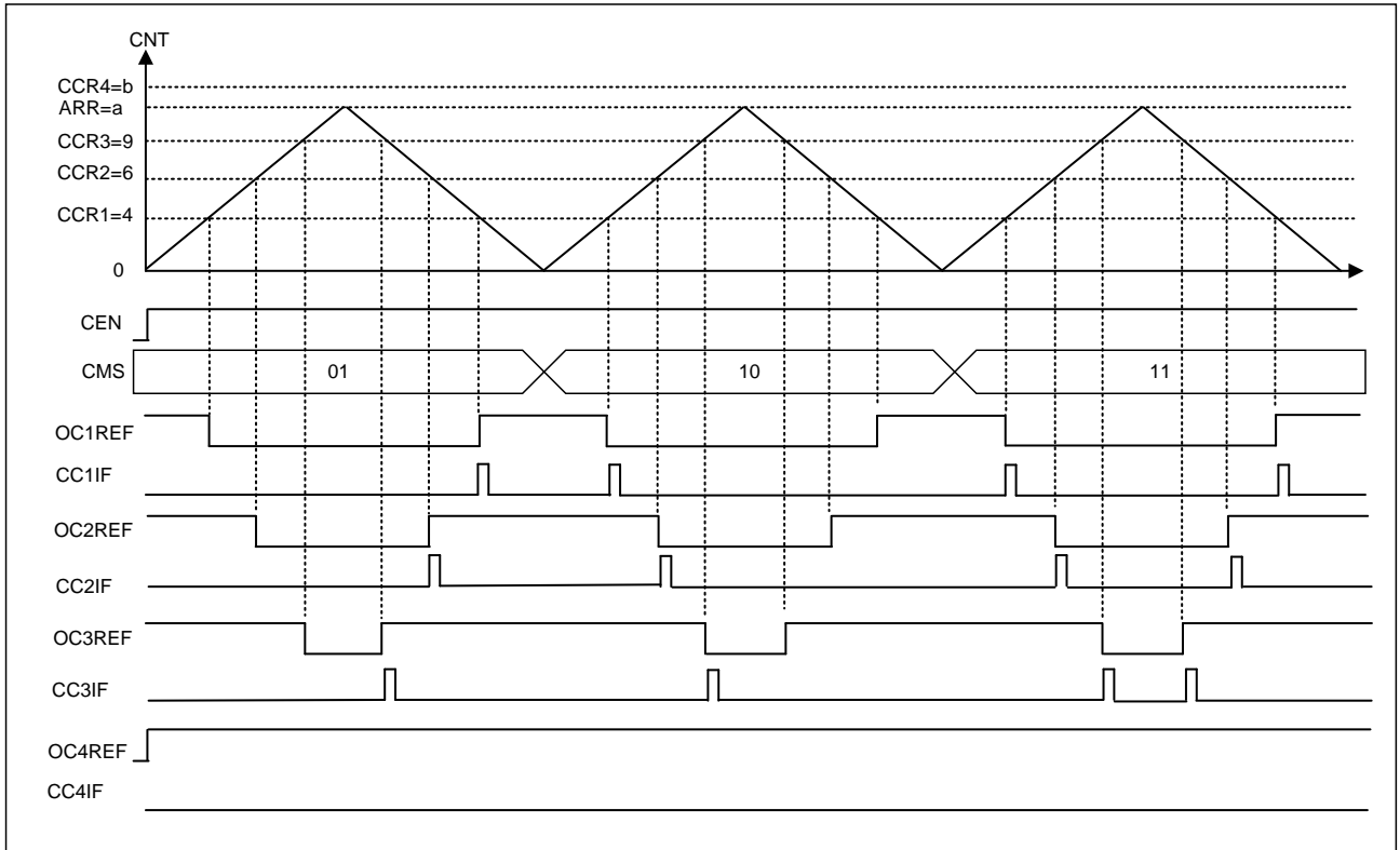
图 15-21 中央对齐 PWM 模式 1 的波形
