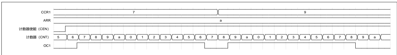
图 19-7 比较输出模式，OC1 信号在匹配时翻转
