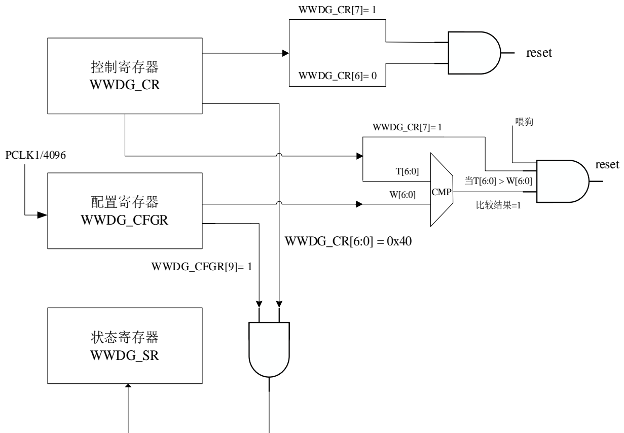
图 20-1 WWDG 功能框图
