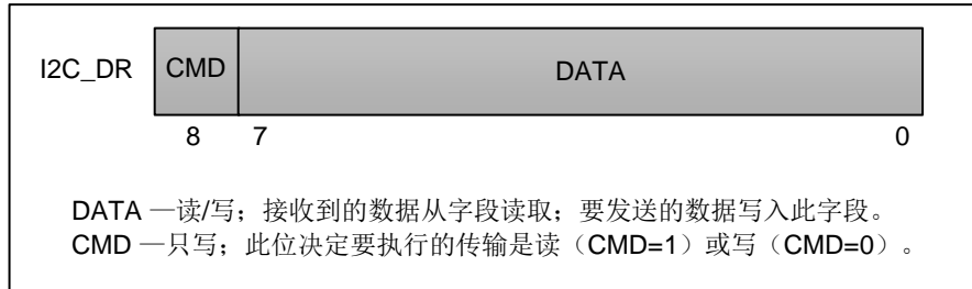
图 25-9 I2C_DR 寄存器
