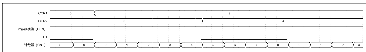
图 17-13 PWM 输入模式时序
