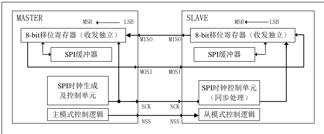
图 24-2 单主和单从应用
