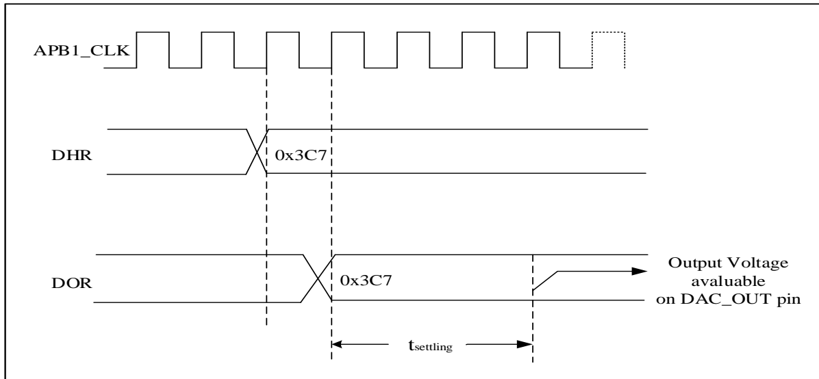
图 14-7 TEN1 = 0 触发关闭时 DAC 转换的时间示意图
