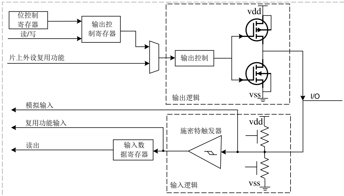
图 9-1 标准 I/O 端口
