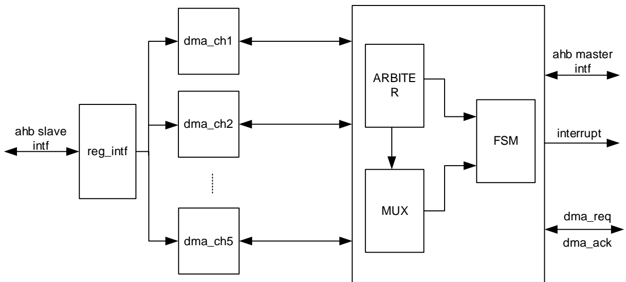
图 11-1 DMA 功能框图
