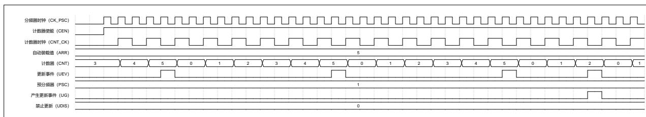
图 19-3 递增计数模式 (UDIS=0)
