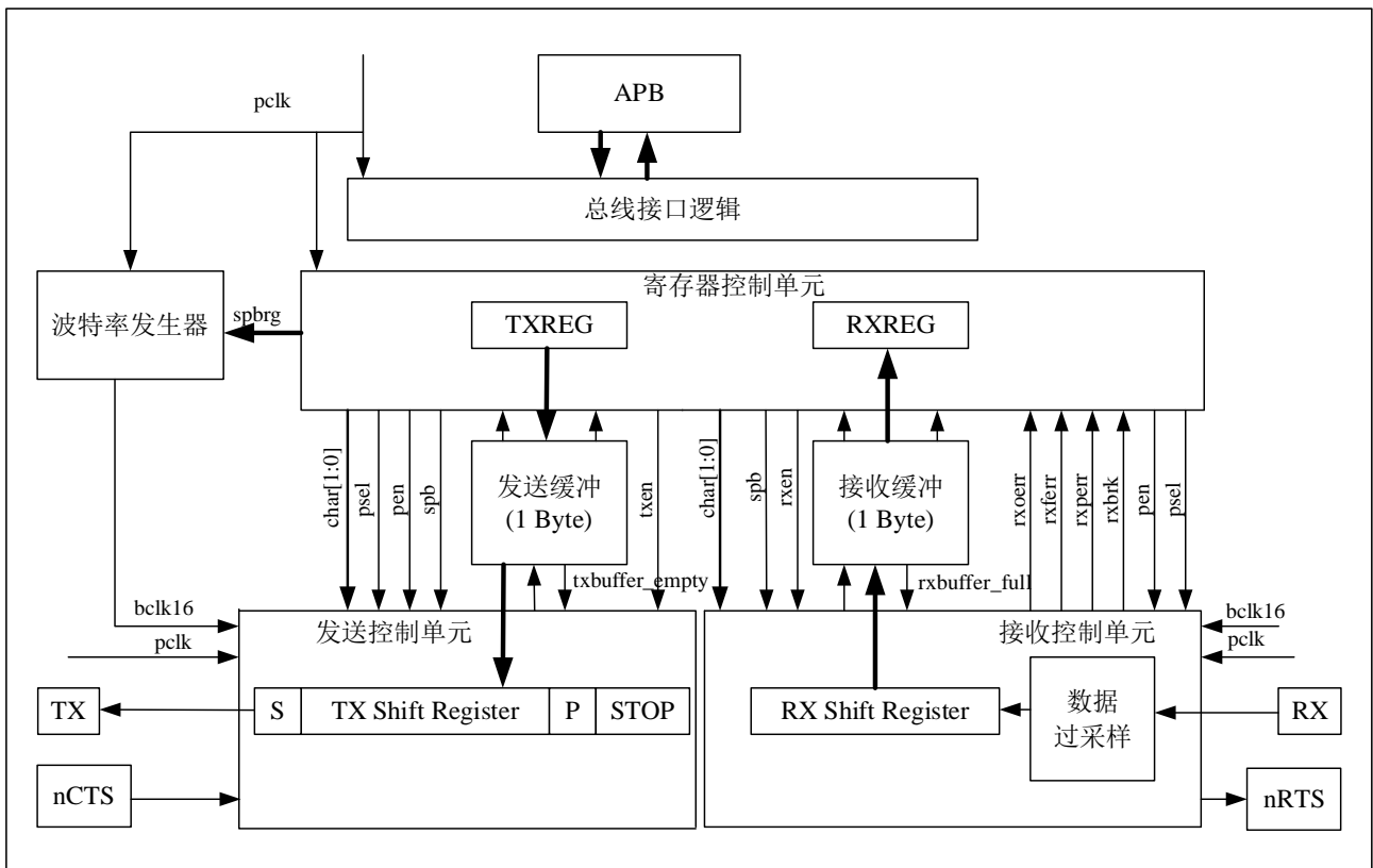
图 23-1 UART 功能框图
