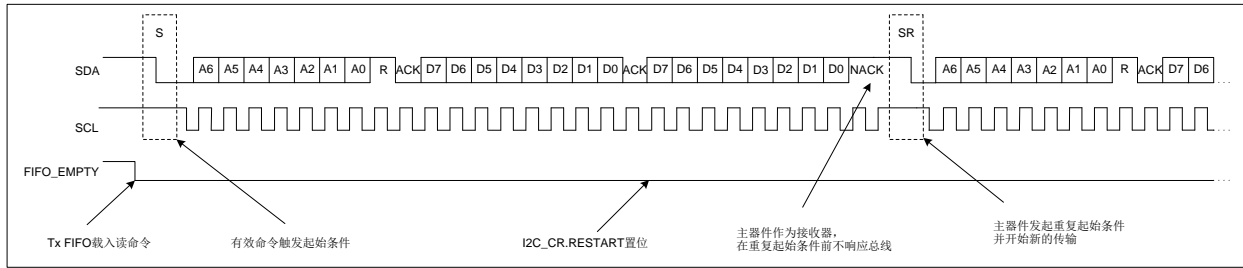
图 25-13 主接收，发生 RESTART
