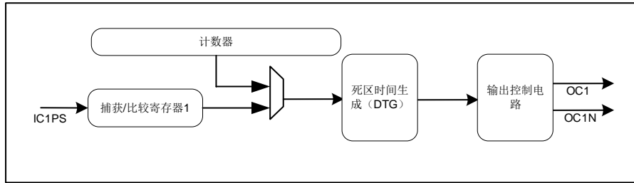
图 19-6 比较输出部分结构图
