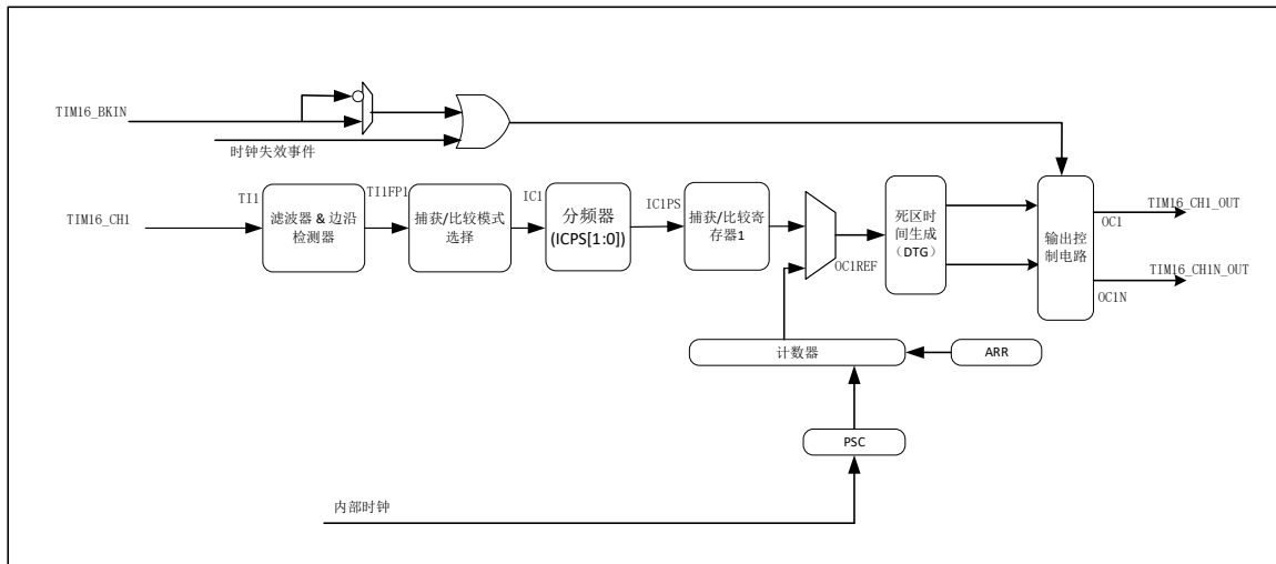
图 19-1 TIMx 结构图
