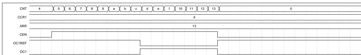
图 18-9 单脉冲模式
