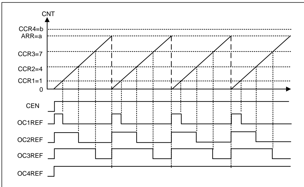
图 16-16 边沿对齐递增计数时 PWM 模式 1 的波形
