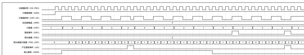
图 15-9 递减计数模式 (UDIS=1 禁止产生更新事件)
