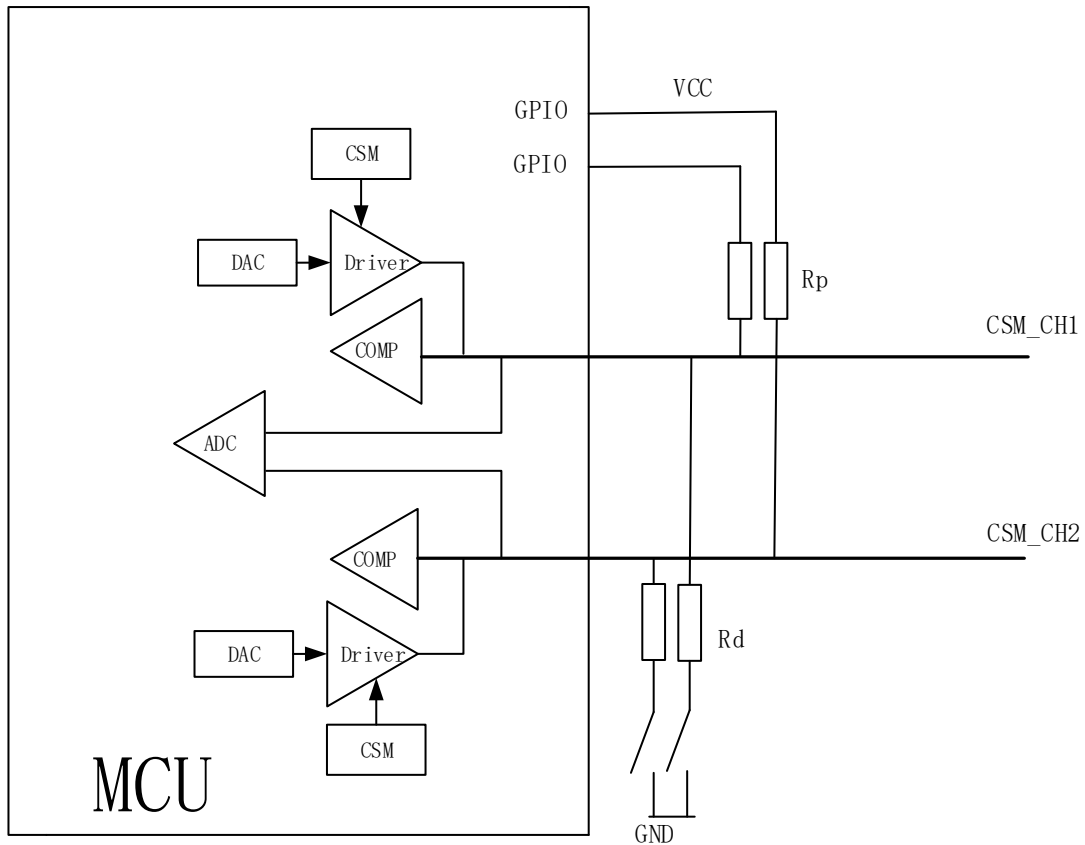
图 26-2 PD 应用示意图
