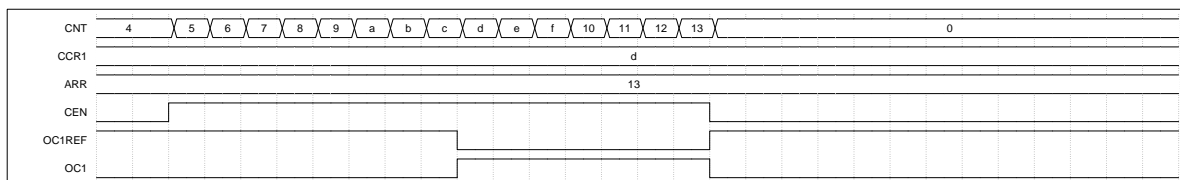
图 19-14 单脉冲模式
