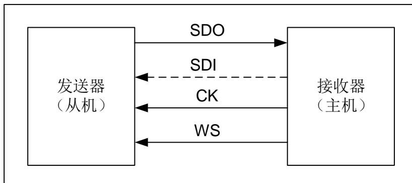
图 24-8 I2S 从模式 (SD 配置成 SDO 为发送器, 配置成 SDI 为接收器)
