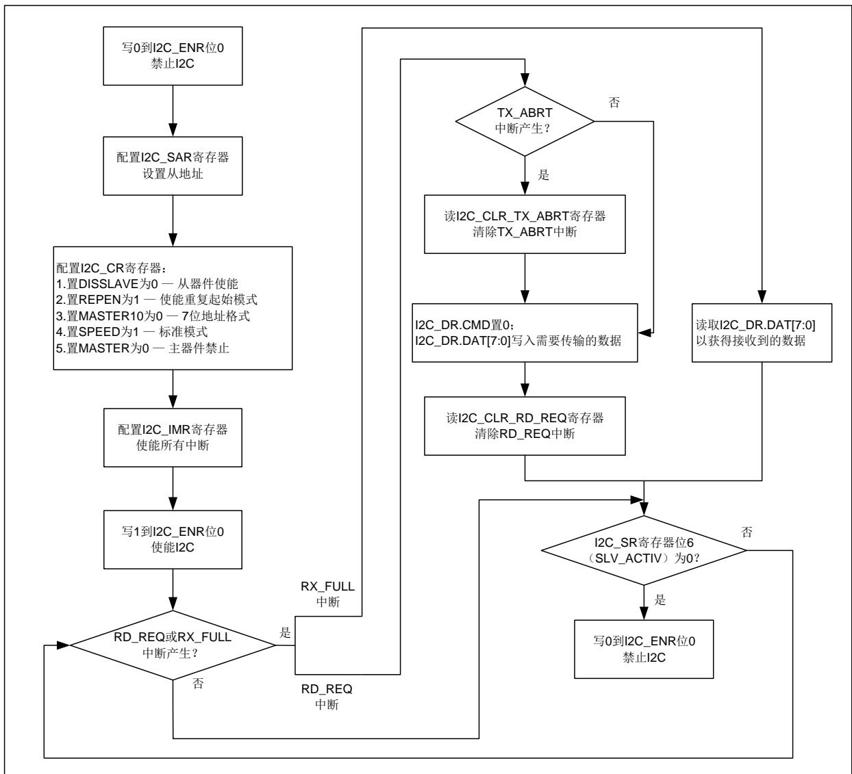
图 25-18 流程图 (I2C 接口作为从器件)
