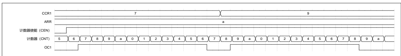
图 16-15 比较输出模式，OC1 信号在匹配时翻转
