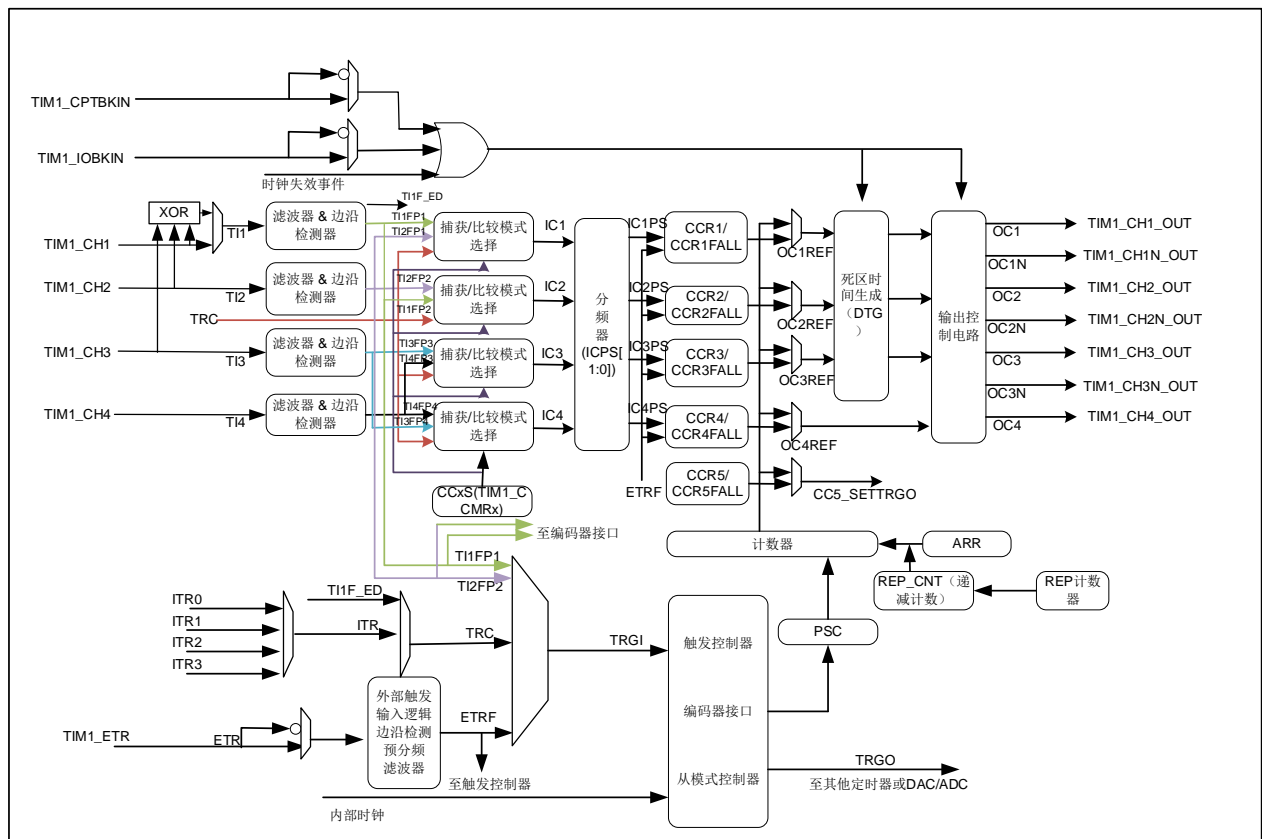
图 15-1 TIMx 结构图
