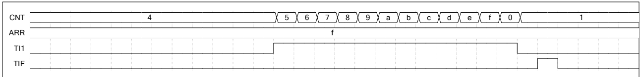
图 15-34 门控模式下的控制时序图
