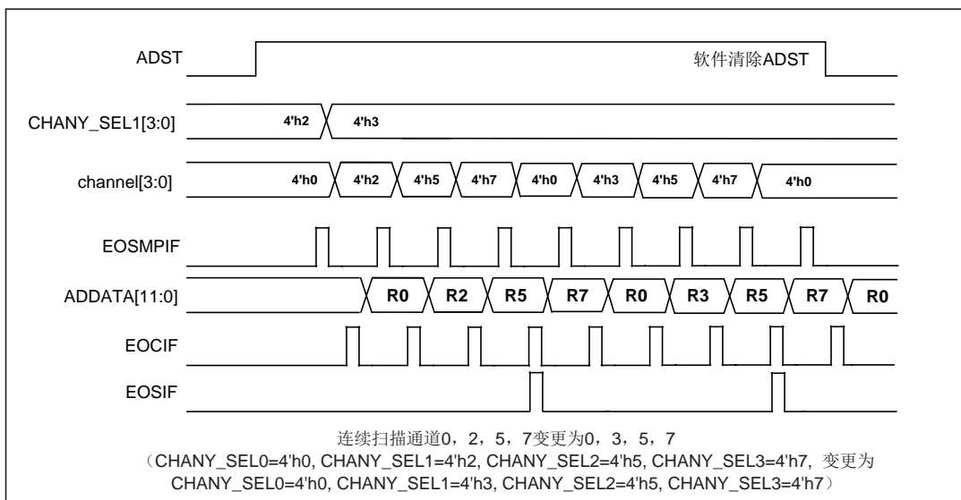
图 13-13 连续扫描模式下动态更新配置时序图
