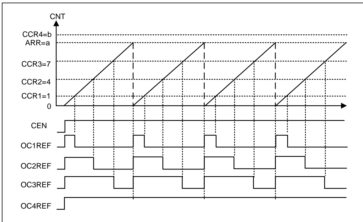
图 17-16 边沿对齐递增计数时 PWM 模式 1 的波形
