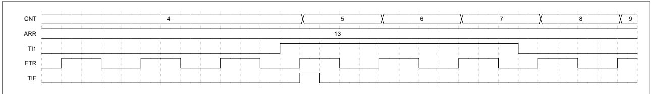
图 17-26 外部时钟模式 2+从模式（触发模式）控制时序图
