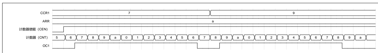
图 18-7 比较输出模式，OC1 信号在匹配时翻转
