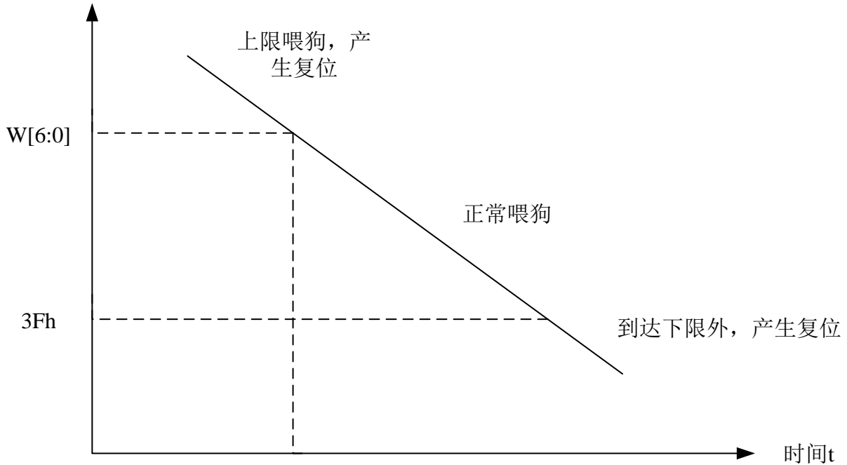
图 20-2 WWDG 超时时间坐标图
