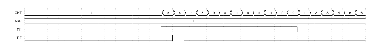
图 15-35 触发器模式下的控制时序图
