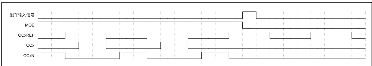
图 15-25 响应刹车的输出（OISx=0, OISxN=0）
