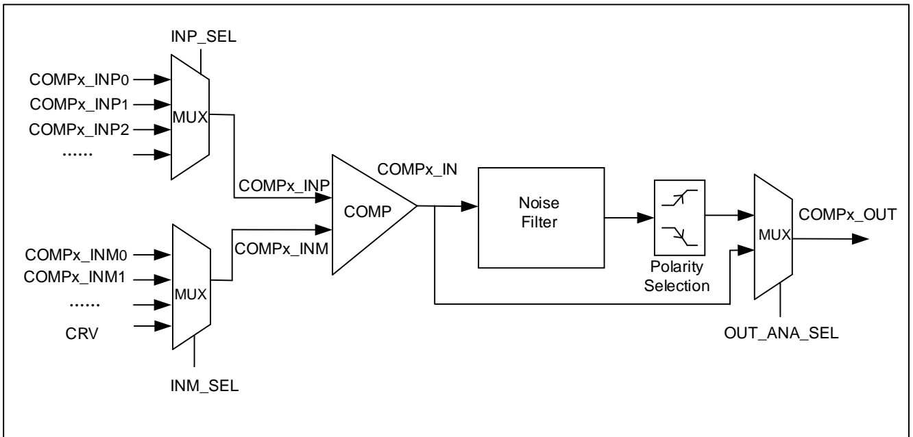
图 12-1 比较器框图
