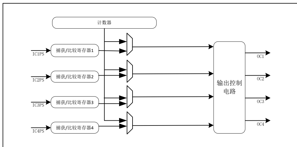
图 16-14 比较输出部分结构图
