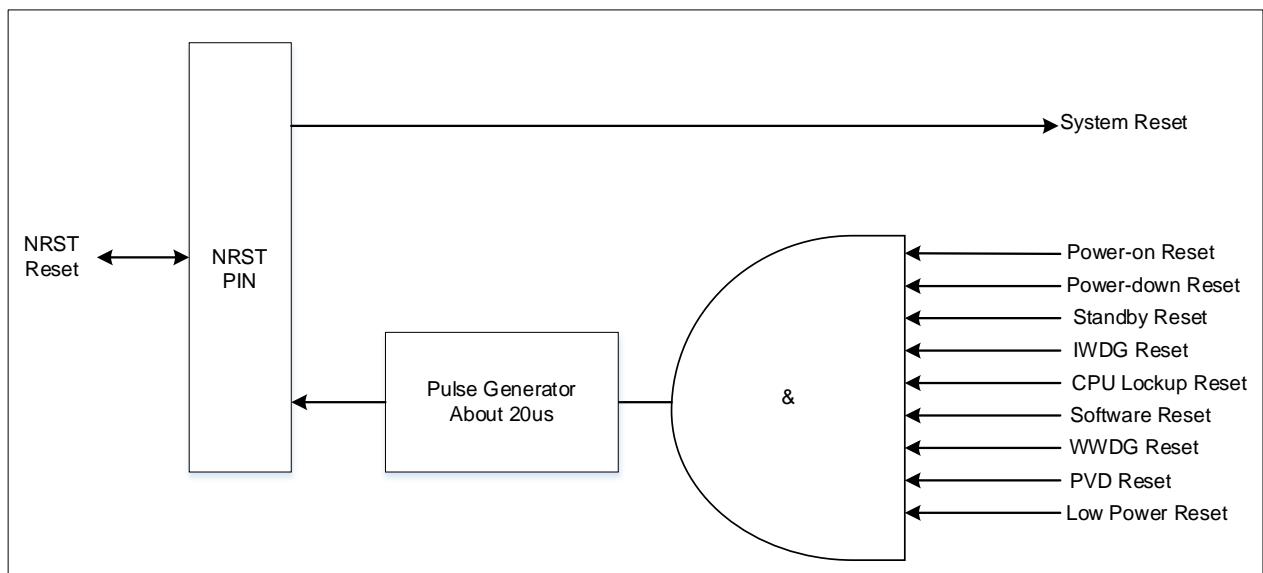
图 5-1 复位功能框图
