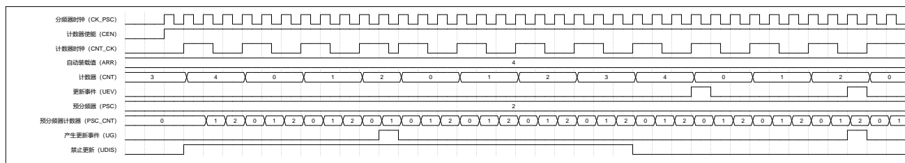
图 15-7 递增计数模式 (UDIS=1 禁止产生更新事件)
