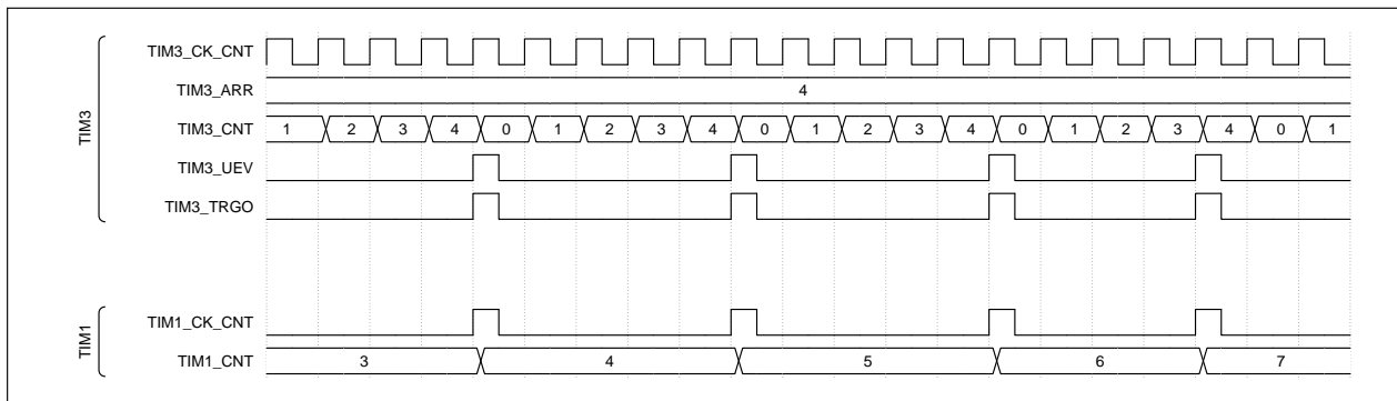
图 15-38 使用 TIM3 作为 TIM1 的预分频器
