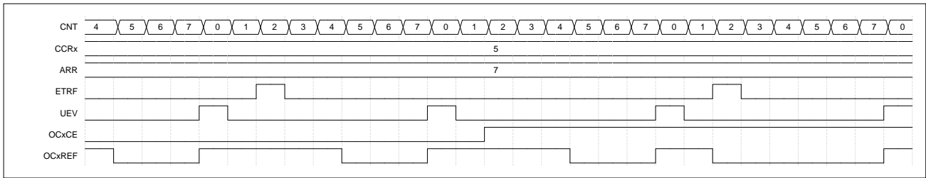
图 17-19 外部事件清除 OCxREF
