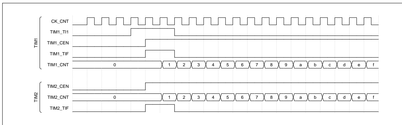
图 15-41 TIM1 的 TI1 同步启动 TIM1 和 TIM2
