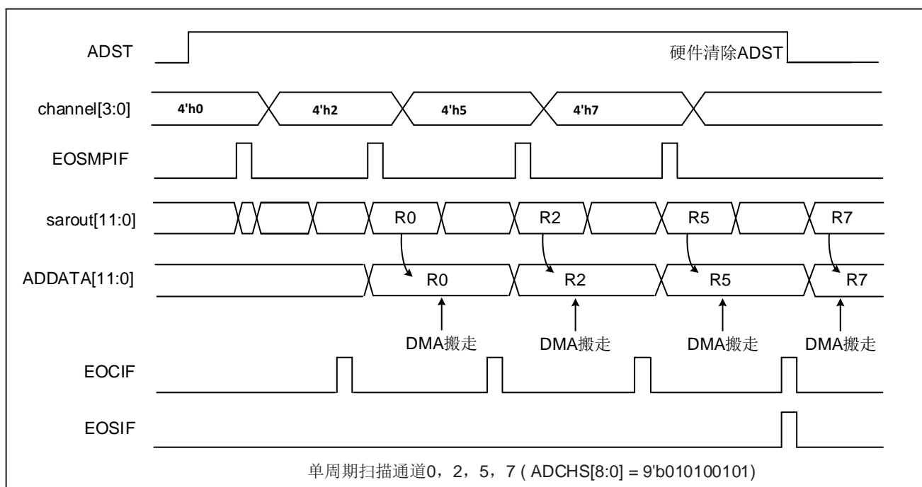
图 13-7 单周期扫描下使能通道转换时序图 (通道方向从高到低)
