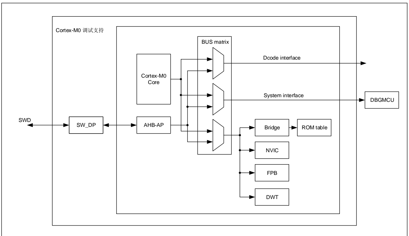
图 28-1 调试功能框图
