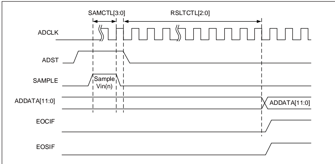
图 13-10 单次转换模式下通道转换时序图
