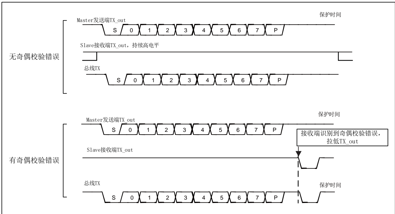
图 23-5 UART 奇偶校验方框图
