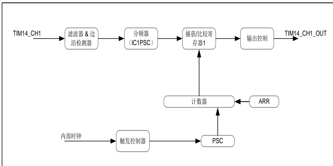
图 18-1 TIM14 结构图
