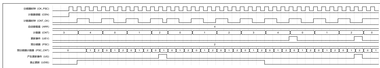
图 19-4 递增计数模式 (UDIS=1 禁止产生更新事件)
