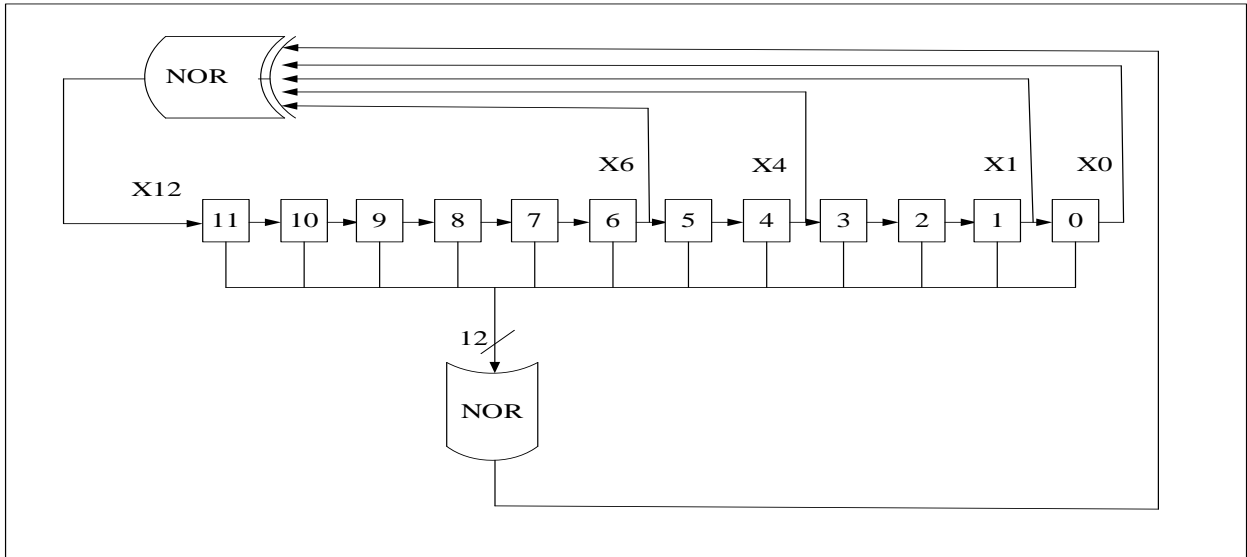
图 14-5 DAC LFSR 寄存器算法
