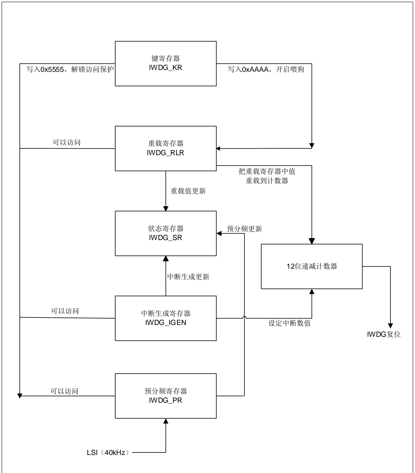
图 21-2 流程框图
