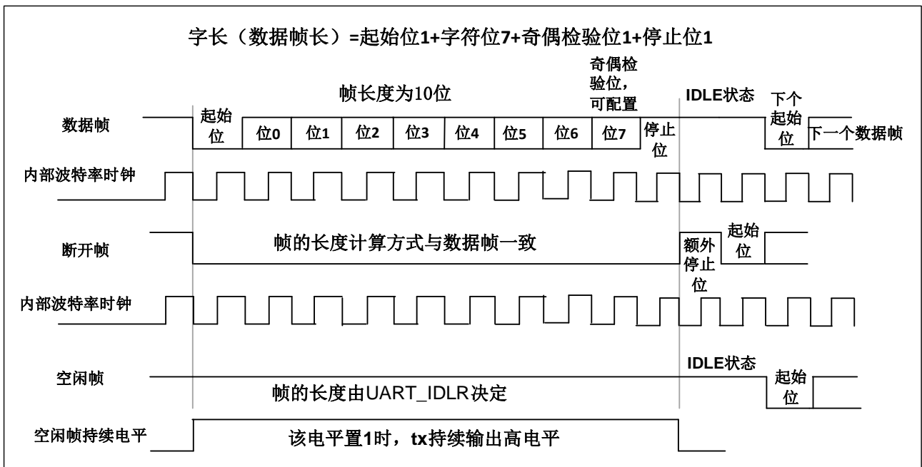
图 23-2 UART 时序
