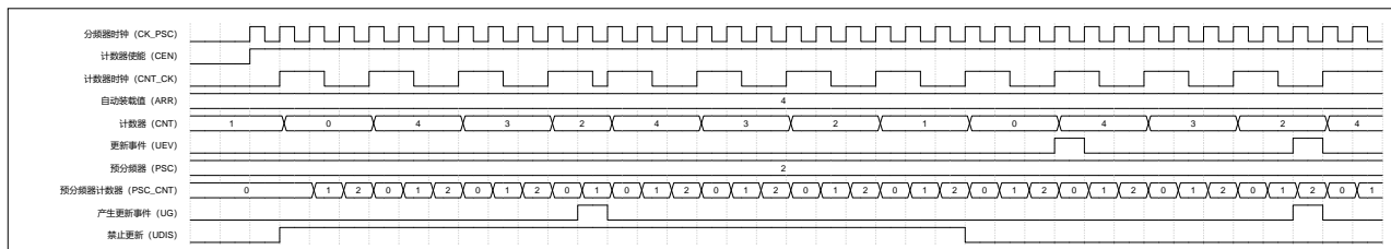
图 16-9 递减计数模式 (UDIS=1 禁止产生更新事件)
