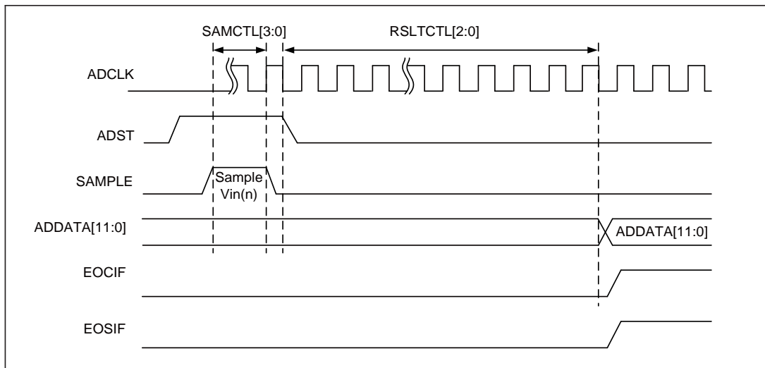
图 13-5 单次转换模式时序图
