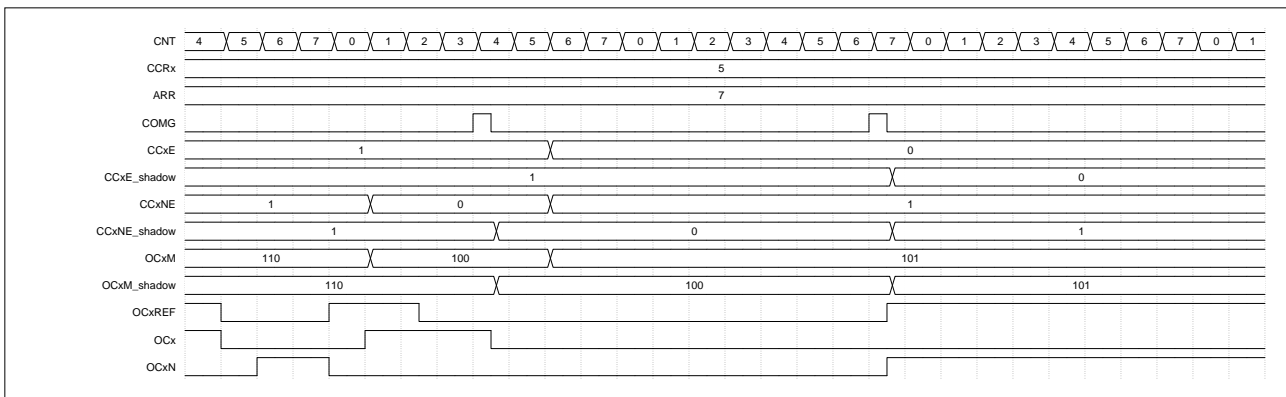
图 15-23 使用 COM 事件产生六步 PWM (OSSR = 1)
