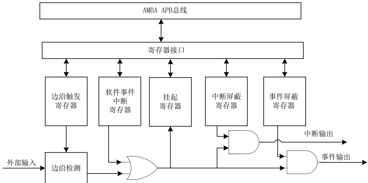
图 10-1 EXTI 结构框图
