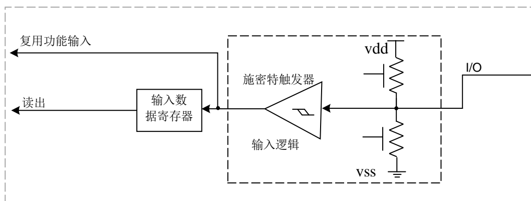
图 9-2 输入浮空/上拉/下拉配置
