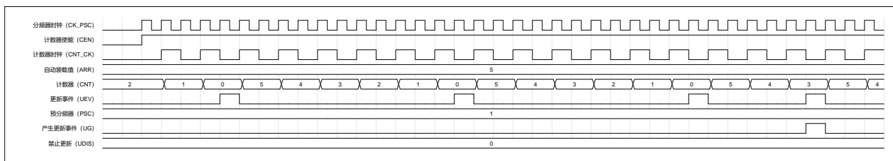
图 16-8 递减计数模式 (UDIS=0)
