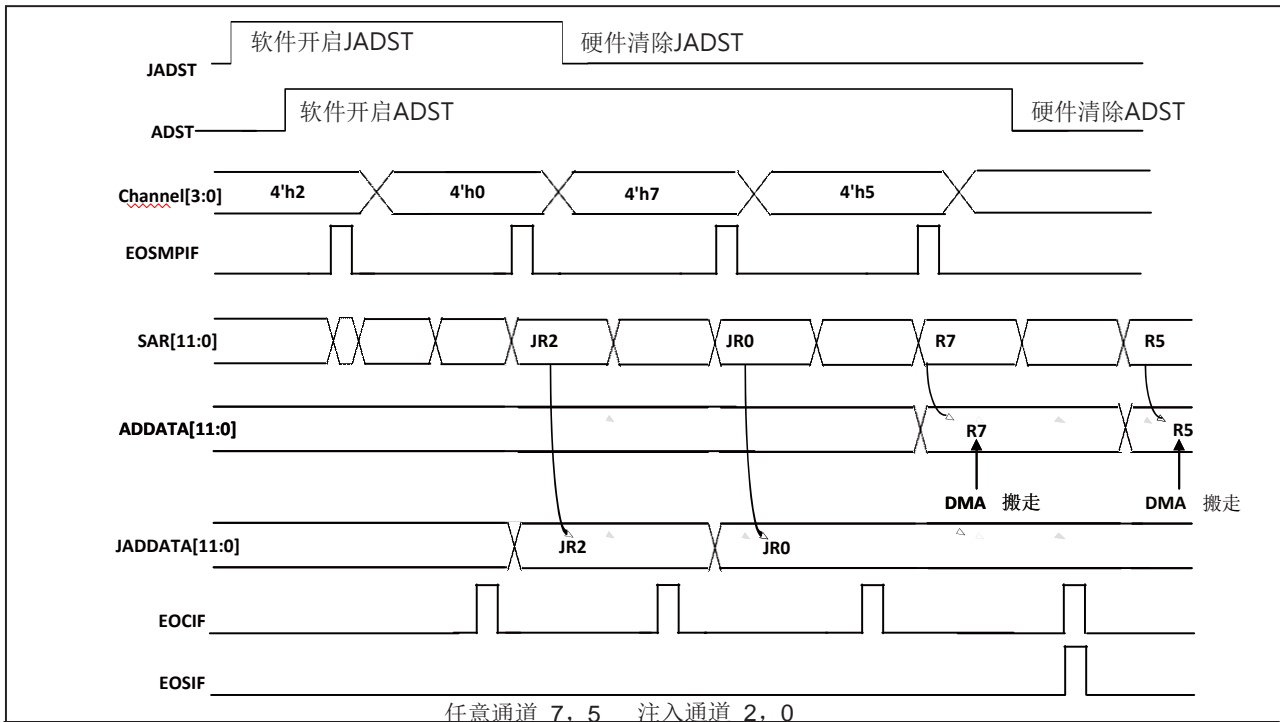
图 13-16 任意通道转换时事件注入通道转换时序图 1
