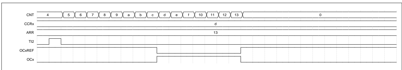
图 16-20 单脉冲模式
