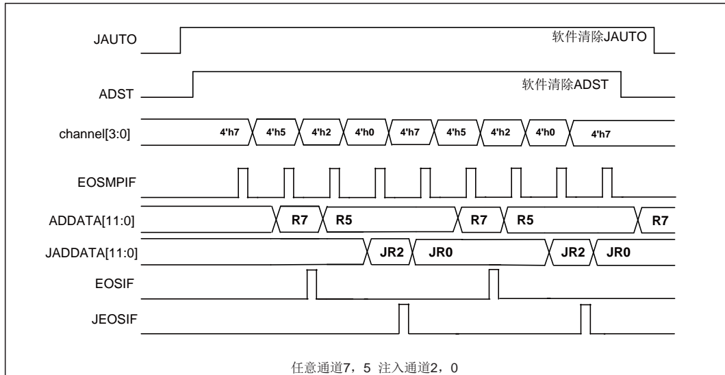
图 13-15 自动注入通道转换连续转换时序图
