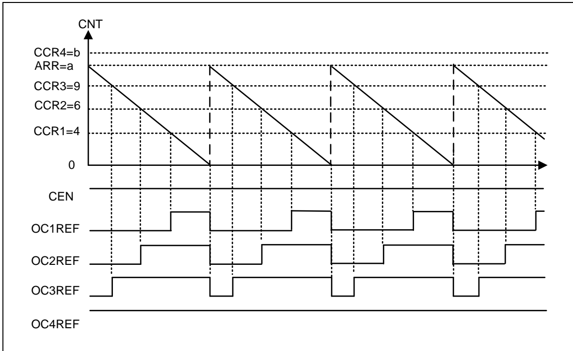
图 16-17 边沿对齐递减计数时 PWM 模式 1 的波形
