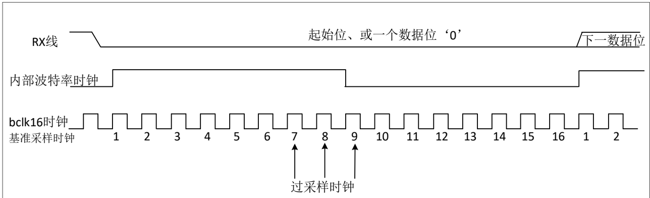
图 23-3 RX 引脚采样方法
