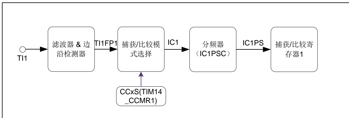
图 18-5 TIM14 输入捕获结构图
