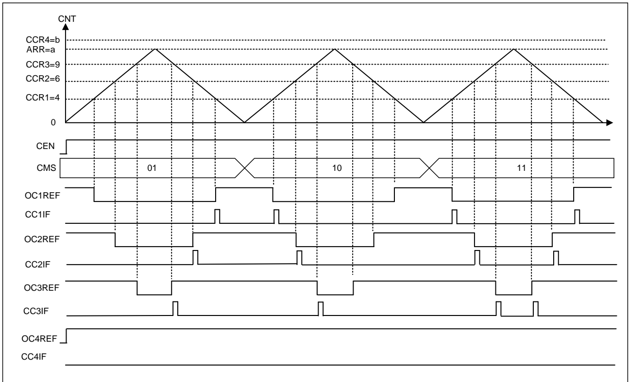
图 17-18 中央对齐 PWM 模式 1 的波形
