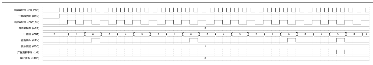
图 17-8 递减计数模式 (UDIS=0)
