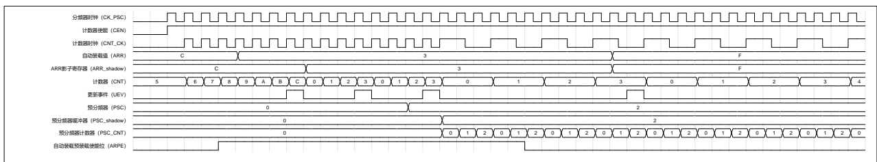
图 18-2 自动预装载
