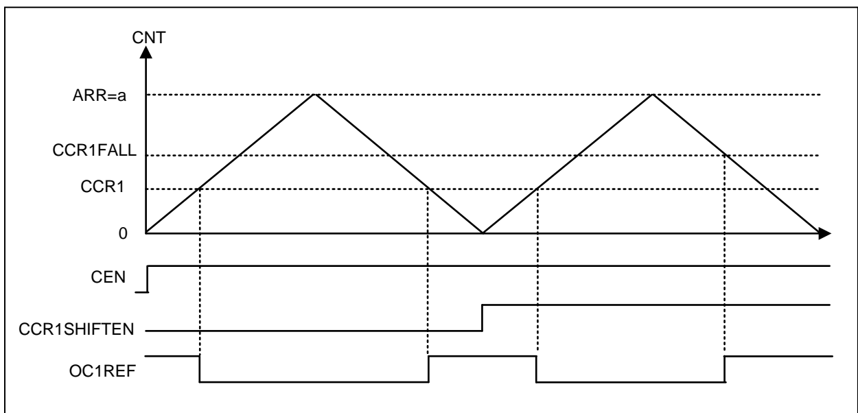
图 15-22 移相功能示意图
