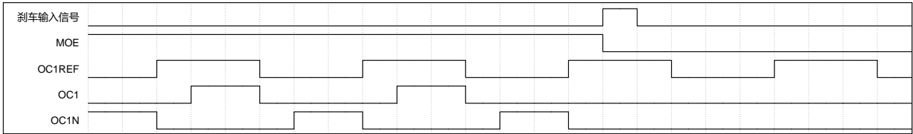
图 19-10 响应刹车的输出 (OISx=0, OISxN=0)
