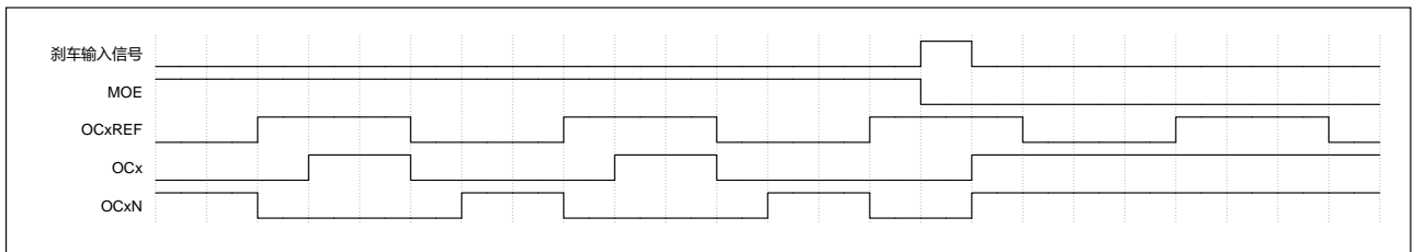
图 15-28 响应刹车的输出（OISx=1, OISxN=1）
