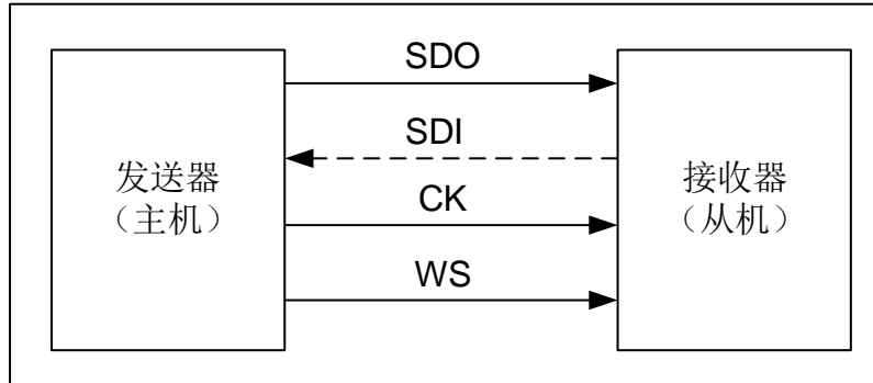
图 24-9 I2S 主模式（SD 配置成 SDO 为发送器，配置成 SDI 为接收器）
