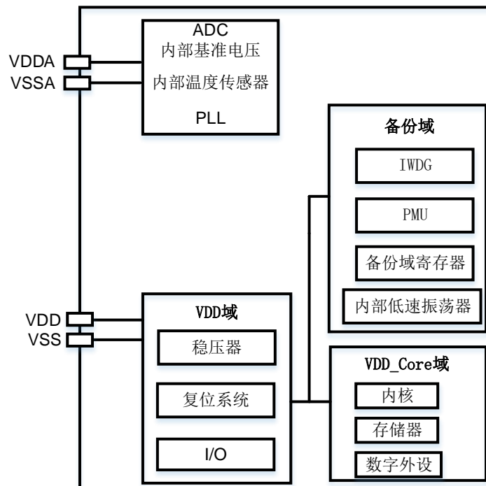
图 3-1 电源控制功能框图
