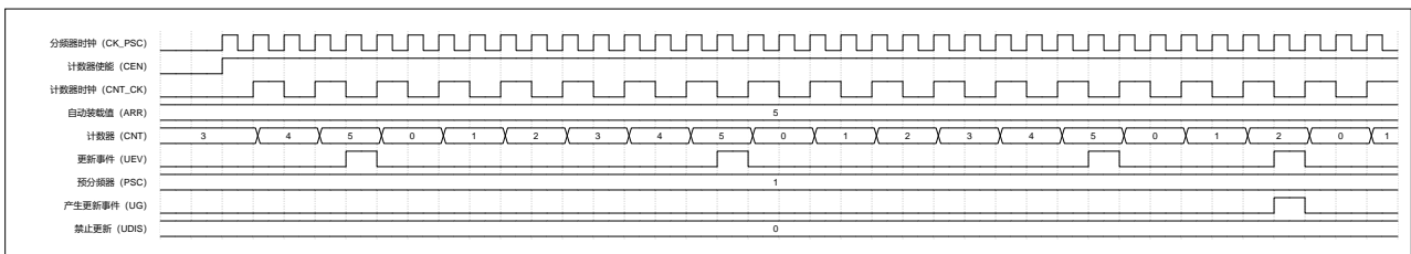
图 16-6 递增计数模式 (UDIS=0)
