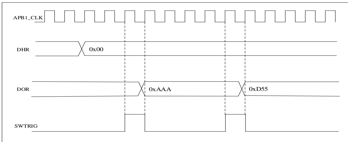
图 14-6 带 LFSR 波形生成的 DAC 转换（使能软件触发）
