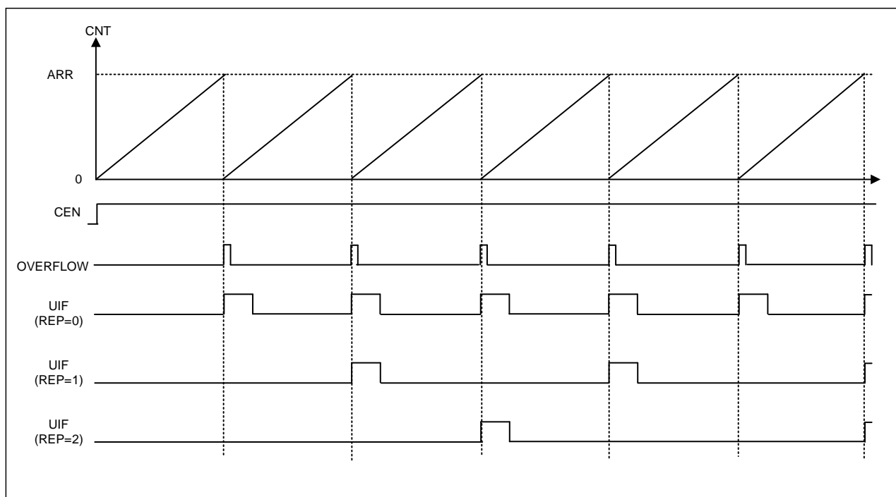
图 15-13 边沿对齐模式递增计数时序图
