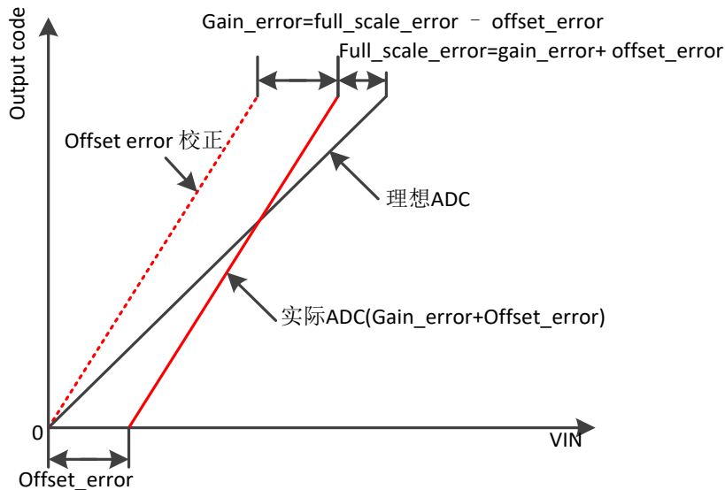
图 13-4 数据误差校正图
