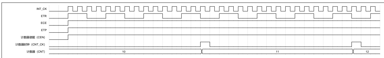
图 15-4 外部时钟模式 2 下的控制电路
