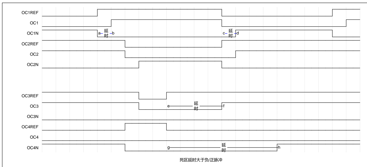
图 15-24 死区插入
