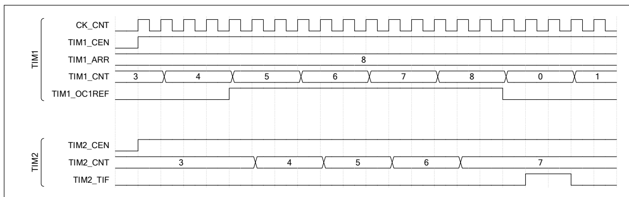
图 15-39 使用 TIM1 使能 TIM2
