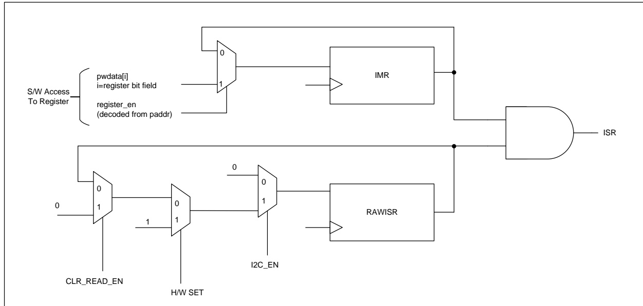
图 25-20 I2C 中断机制
