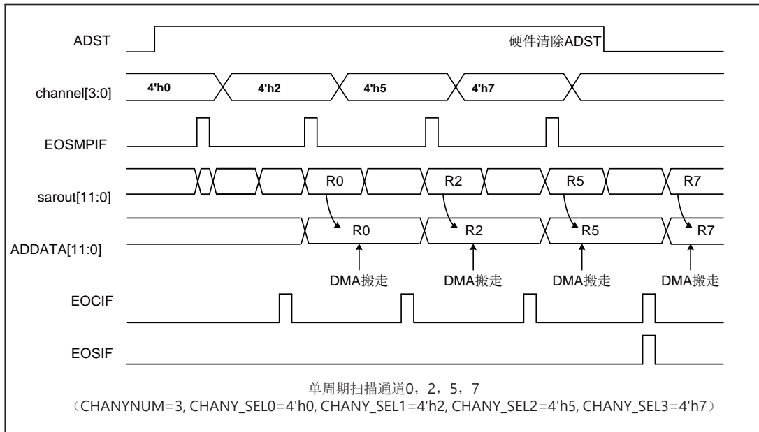
图 13-11 单周期扫描下通道转换时序图
