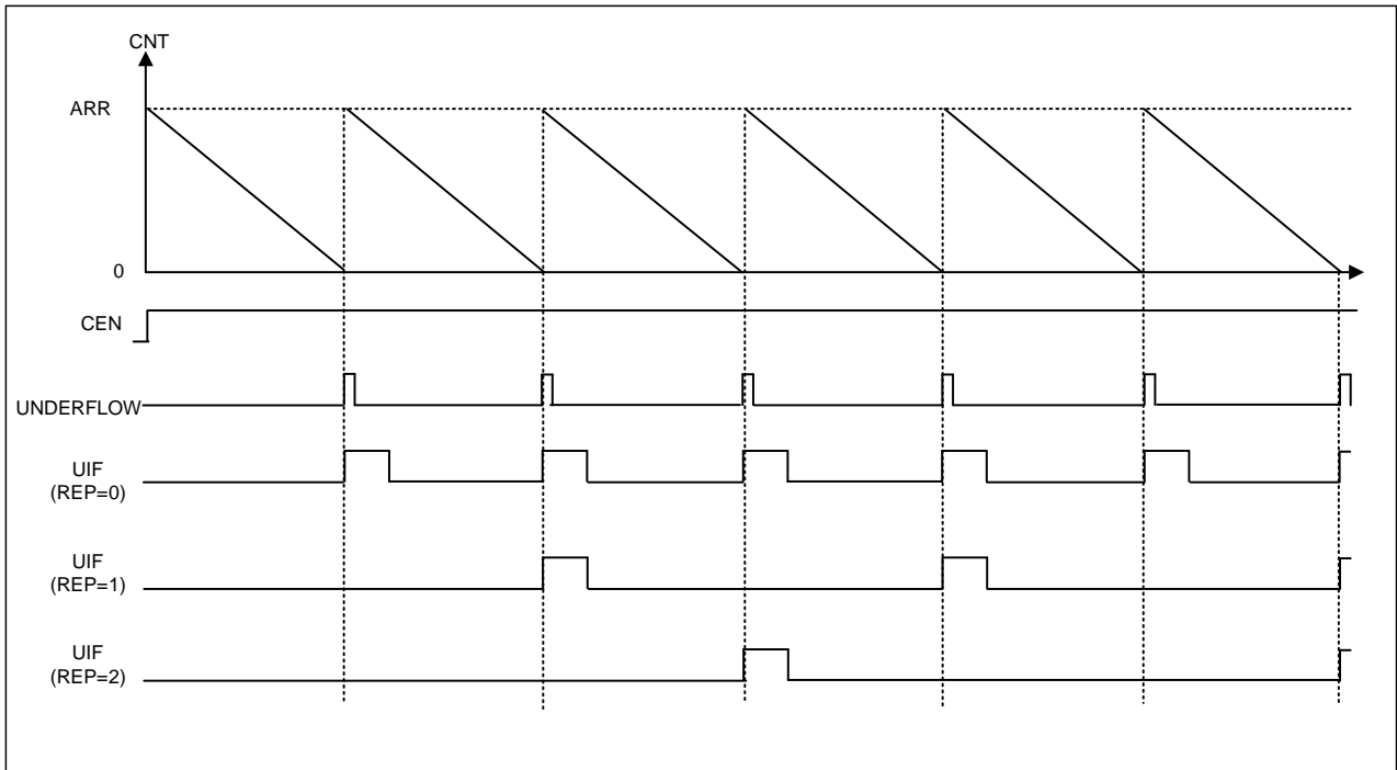
图 15-14 边沿对齐模式递减计数时序图
