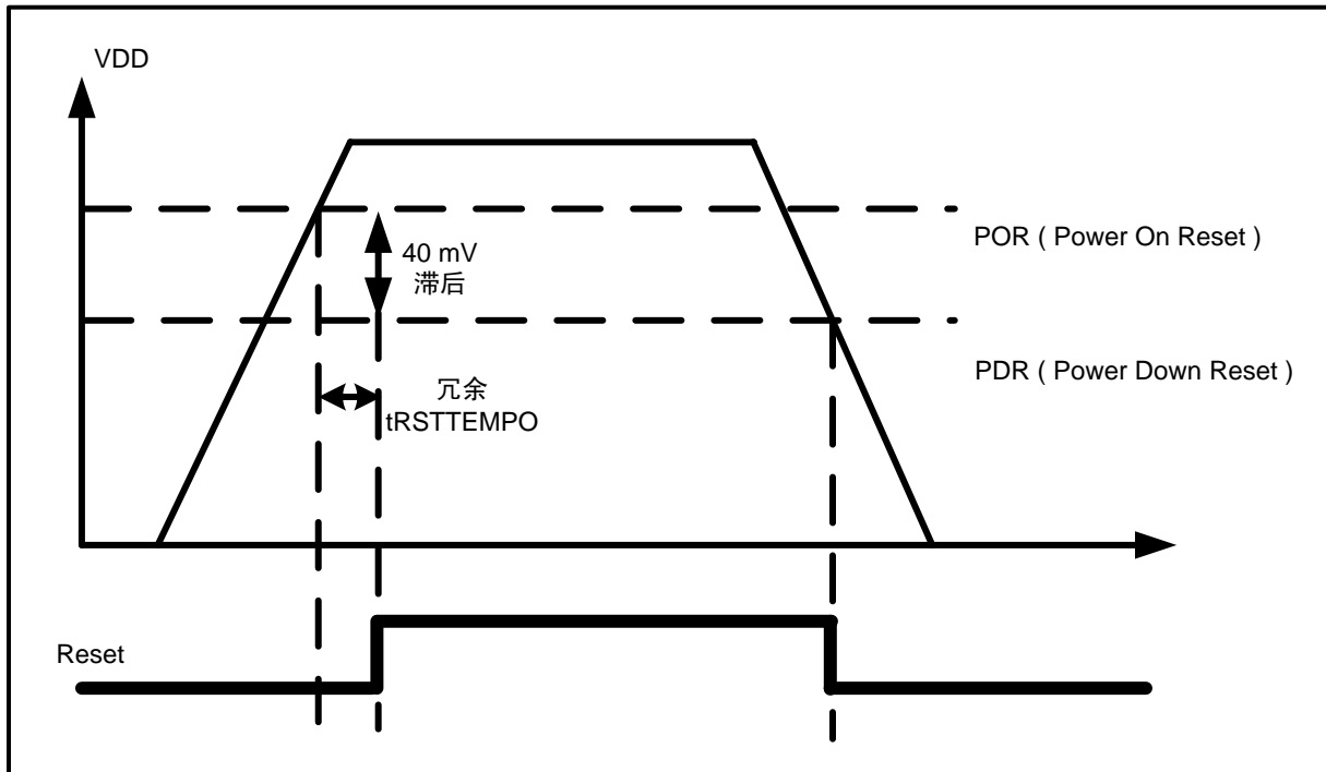
图 3-2 上电复位和掉电复位波形图
