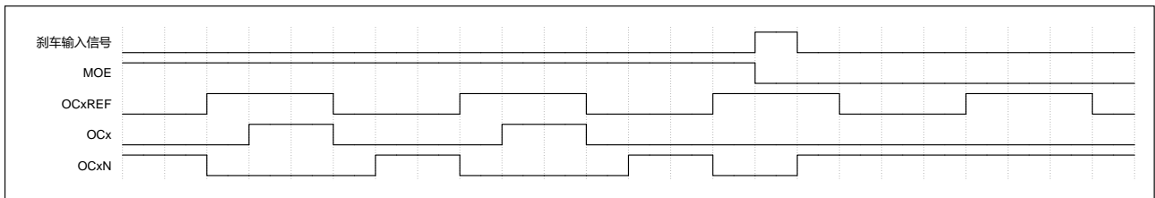
图 15-26 响应刹车的输出（OISx=0, OISxN=1）
