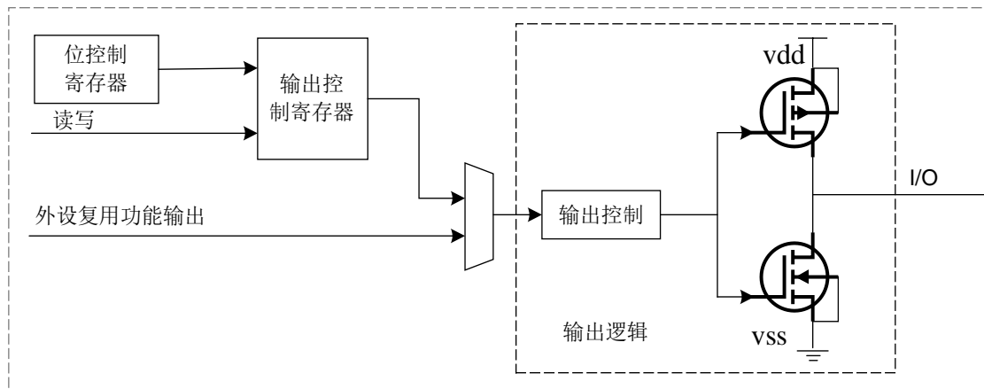
图 9-3 输出配置
