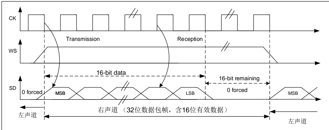
图 24-5 MSB 对齐标准示意图
