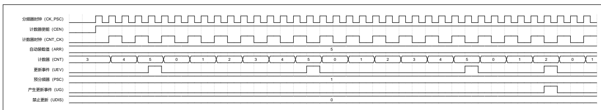
图 18-3 递增计数模式（UDIS=0）
