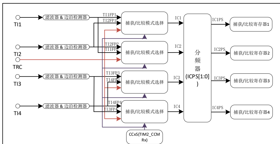
图 16-12 TIM2 输入捕获结构图
