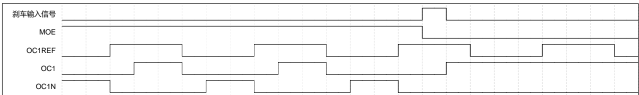
图 19-12 响应刹车的输出 (OISx=1, OISxN=0)
