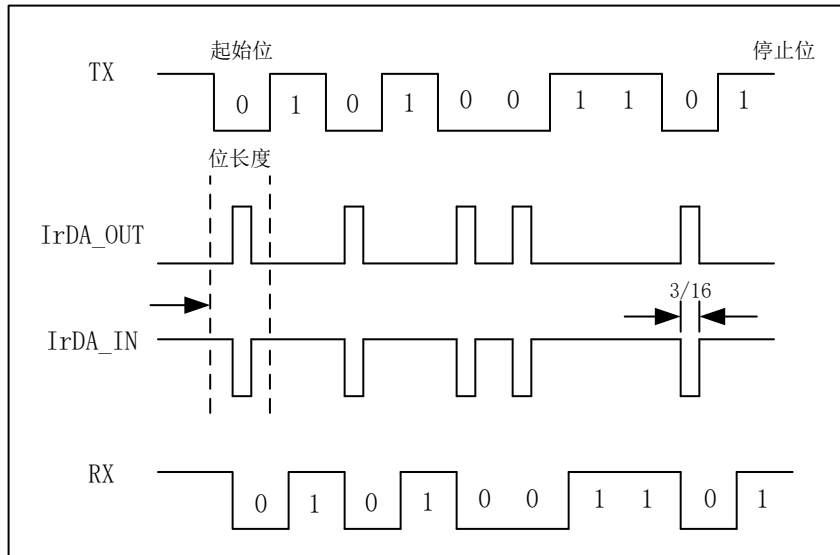
图 23-7 普通模式下 IrDA 发送和接收图
