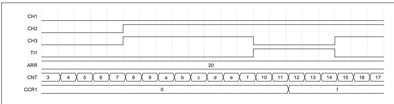
图 15-42 (TI1 异或输入) 输入捕获波形图
