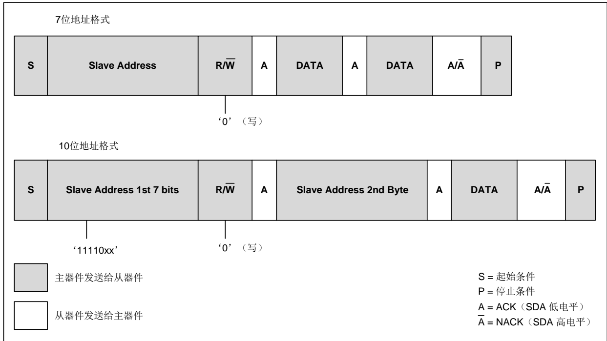
图 25-5 主发送协议
