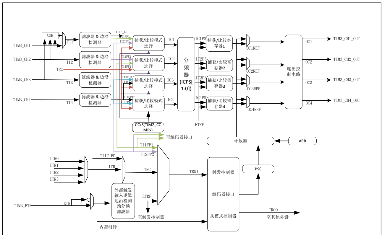
图 17-1 TIM3 结构图
