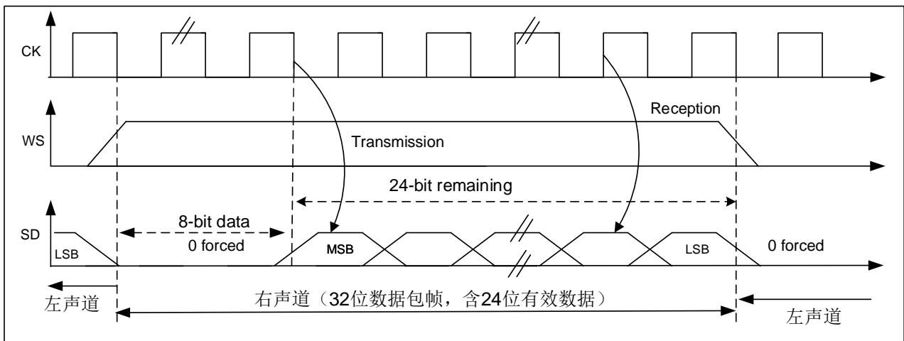
图 24-6 LSB 对齐标准示意图
