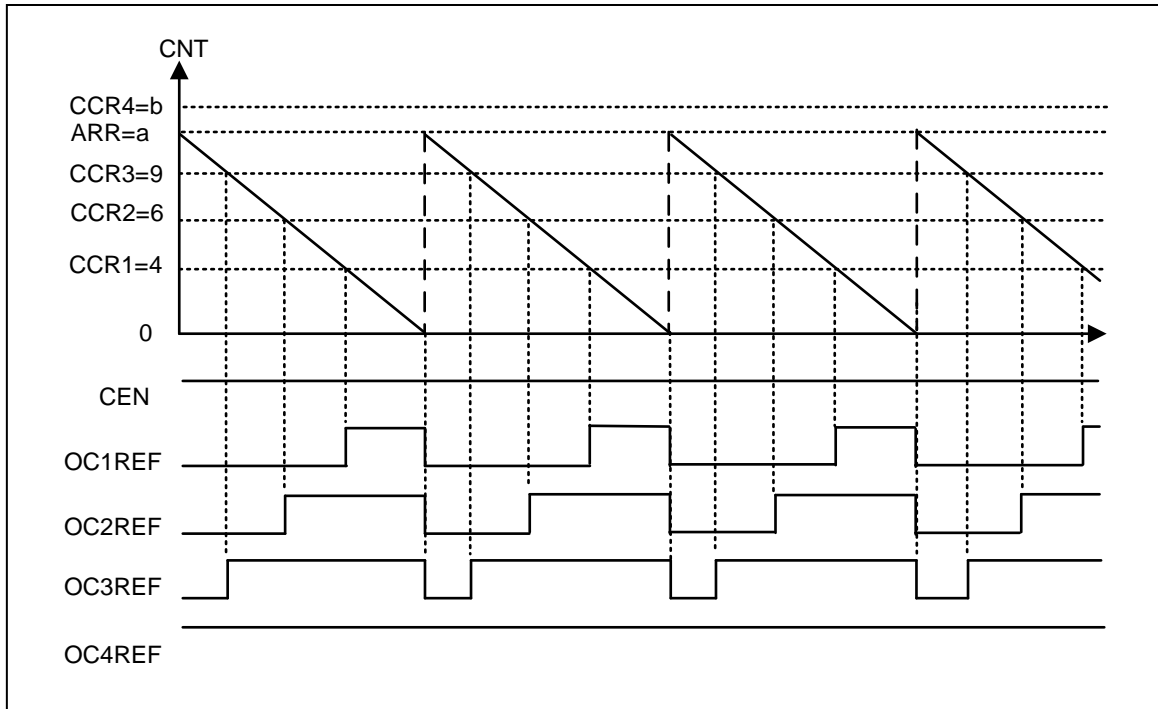
图 17-17 边沿对齐递减计数时 PWM 模式 1 的波形
