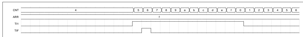
图 17-25 触发器模式下的控制时序图
