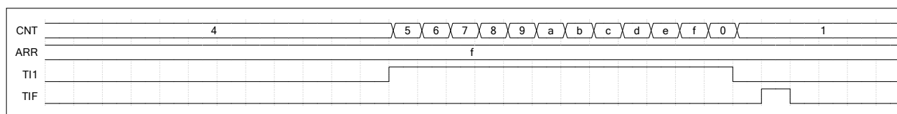
图 17-24 门控模式下的控制时序图
