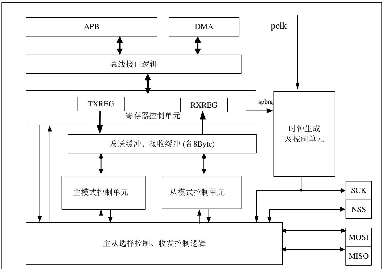
图 24-1 SPI_I2S 功能框图
