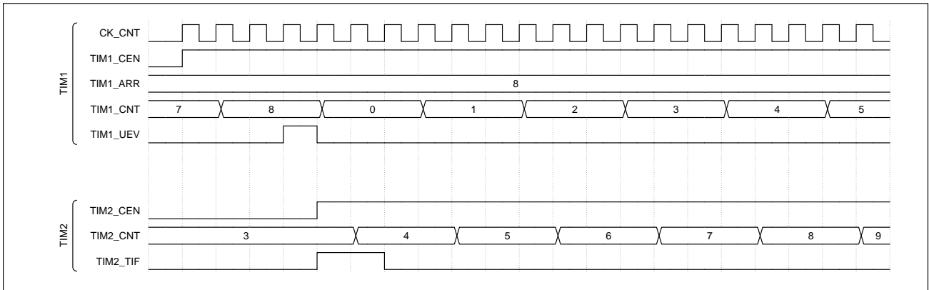
图 15-40 使用 TIM1 的更新事件启动 TIM2
