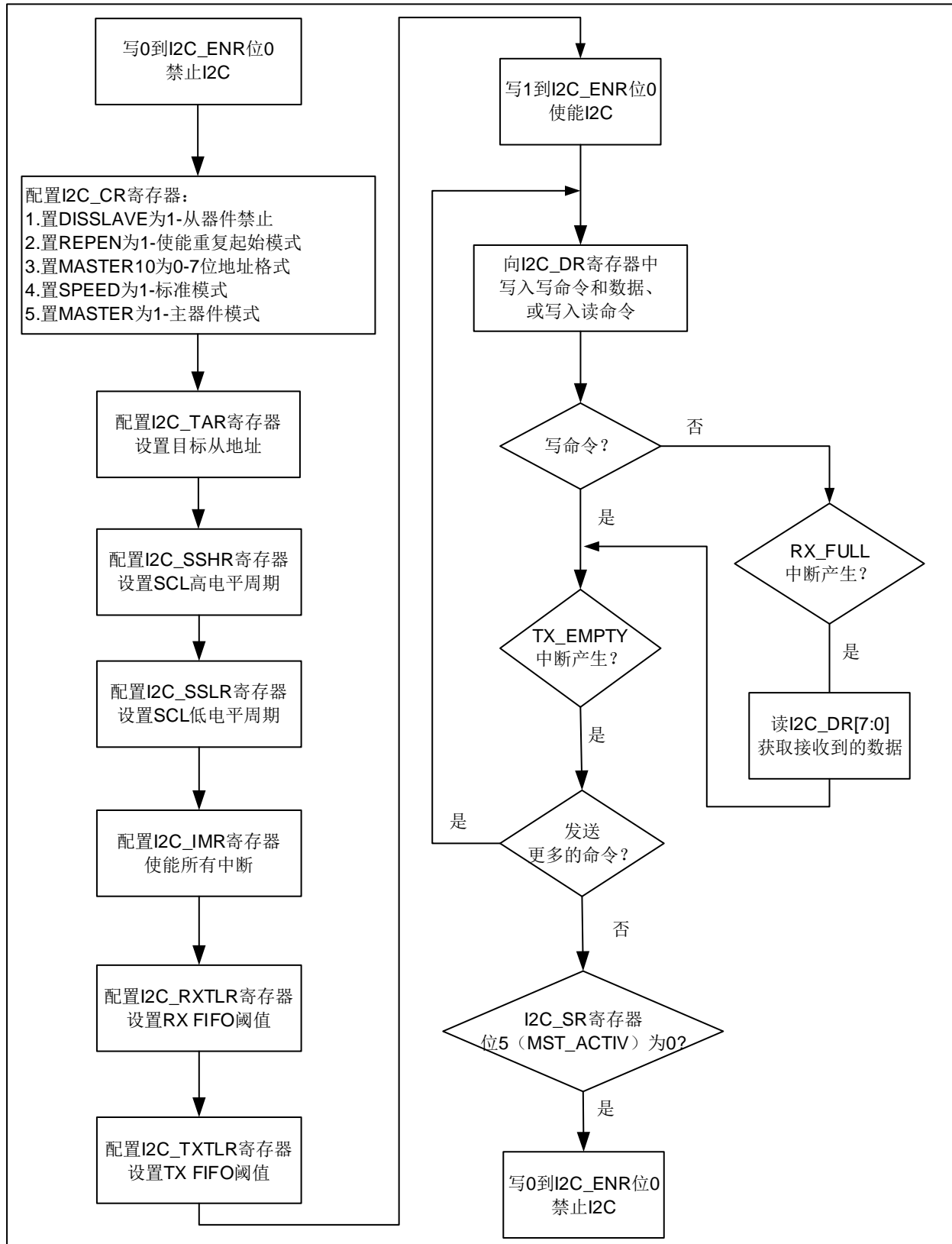
图 25-19 流程图 (I2C 接口作为主器件)
