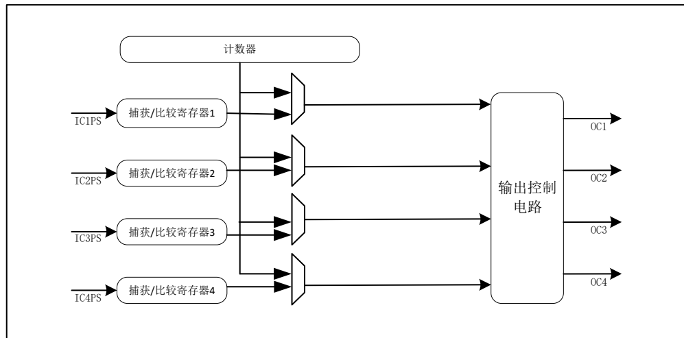
图 17-14 比较输出部分结构图
