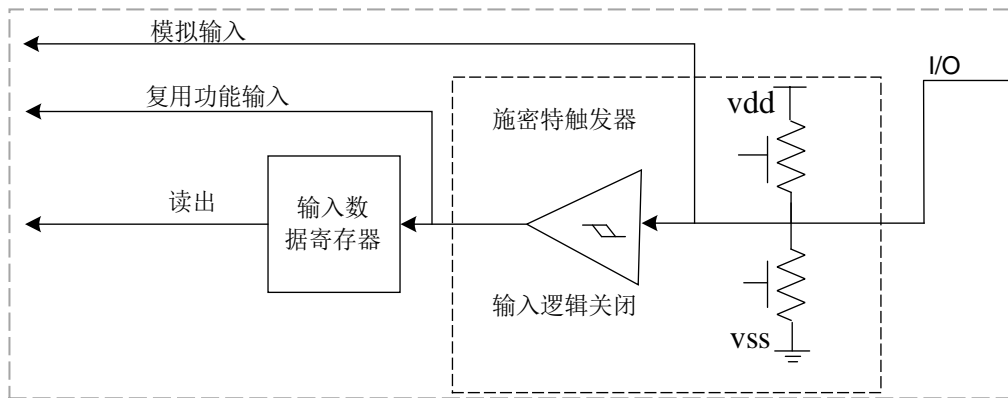
图 9-5 模拟输入
