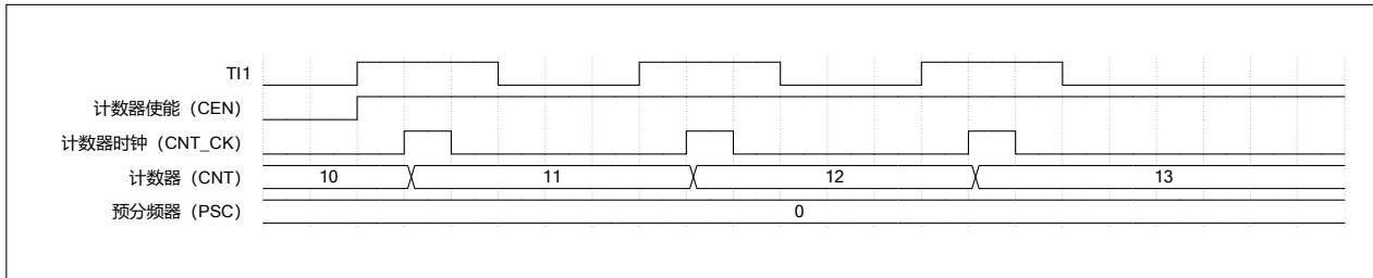
图 15-3 外部时钟模式 1 下的控制电路
