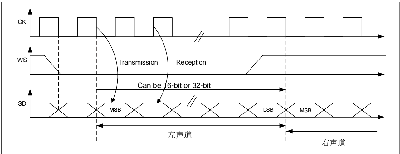
图 24-4 飞利浦标准示意图
