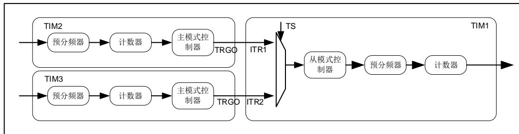
图 15-37 定时器间互联
