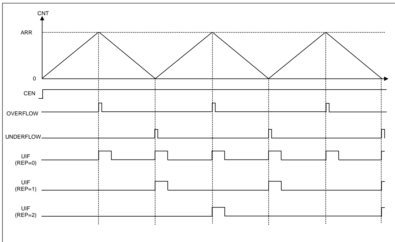
图 15-12 中央对齐模式重复计数时序图
