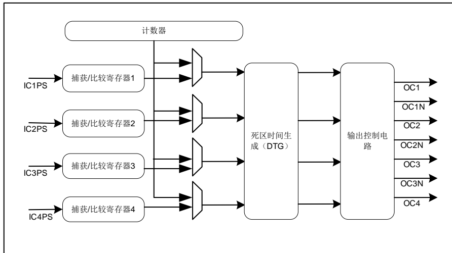
图 15-17 比较输出部分结构图
