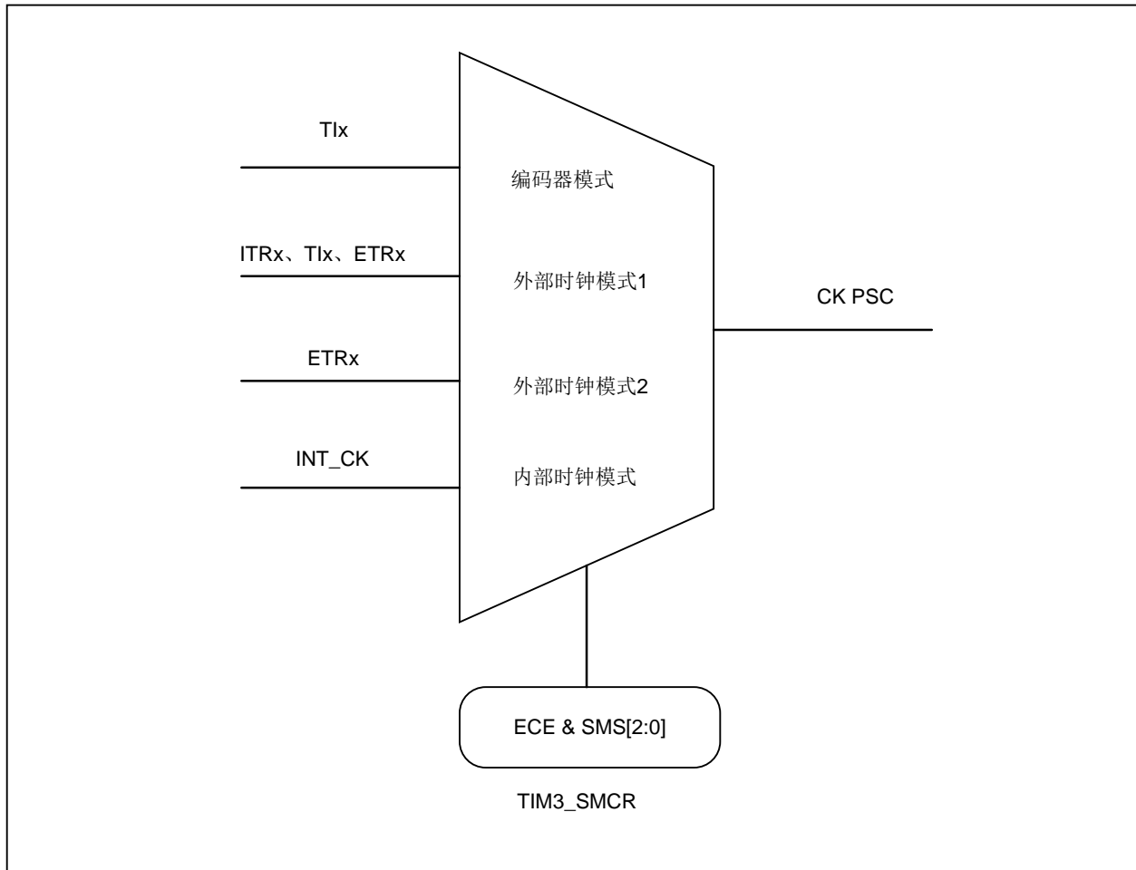
图 17-2 时钟选择
