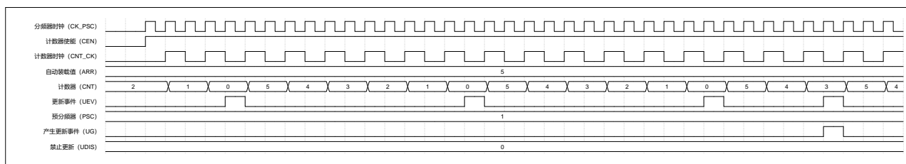
图 15-8 递减计数模式 (UDIS=0)
