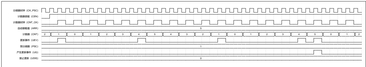
图 17-10 中央计数模式（UDIS=0）
