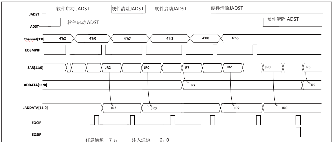
图 13-17 任意通道转换时事件注入通道转换时序图 2
