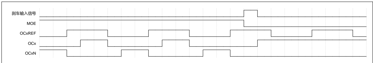
图 15-27 响应刹车的输出（OISx=1, OISxN=0）
