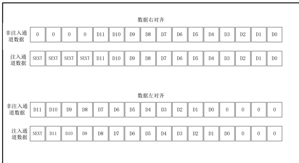
图 13-2 数据对齐方式
