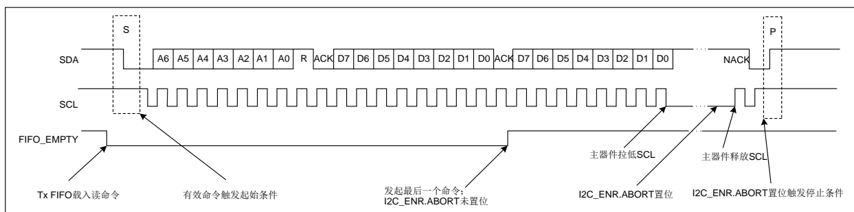
图 25-11 主接收，TX FIFO 为空
