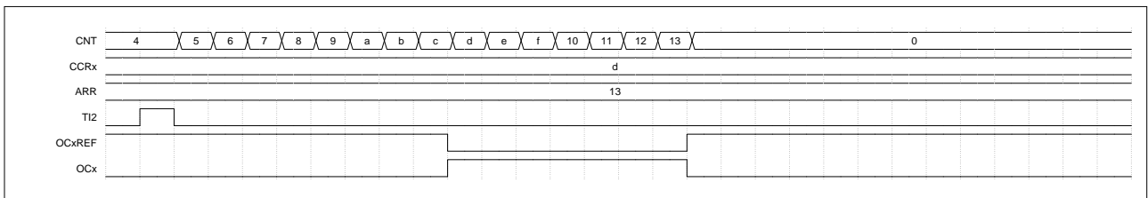
图 15-30 单脉冲模式
