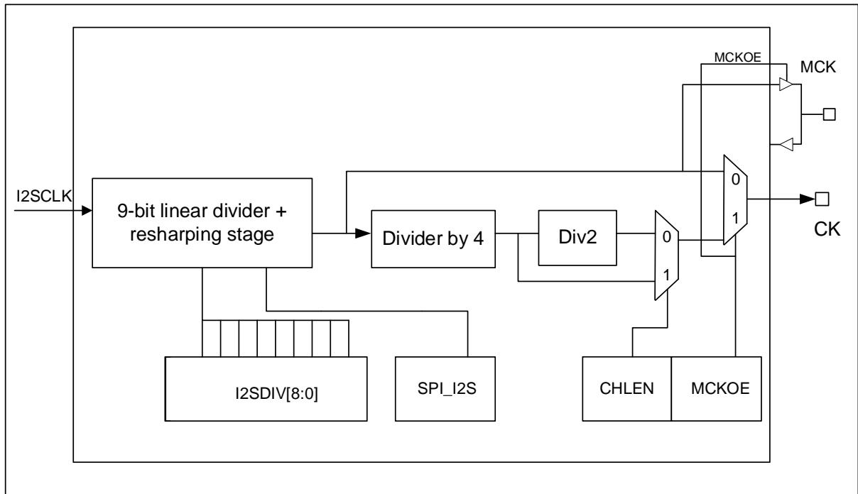
图 24-10 I2S 时钟预分频器示意图
