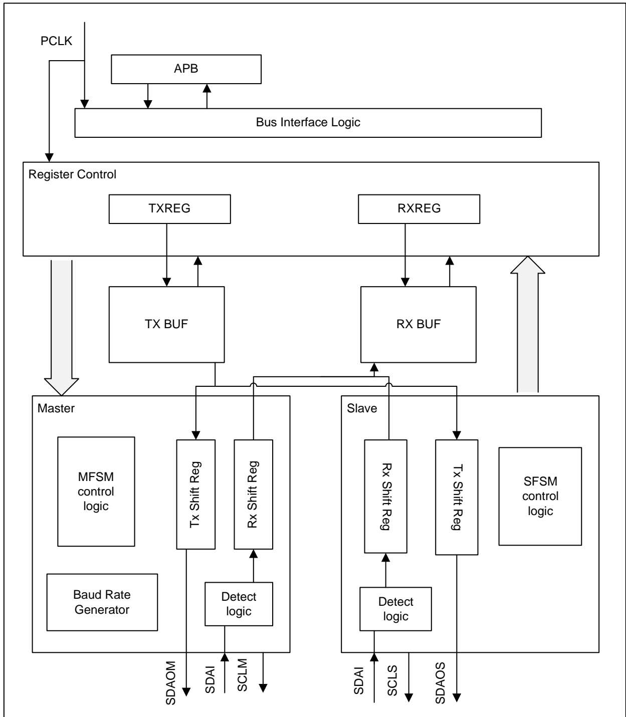
图 25-1 I2C 功能框图
