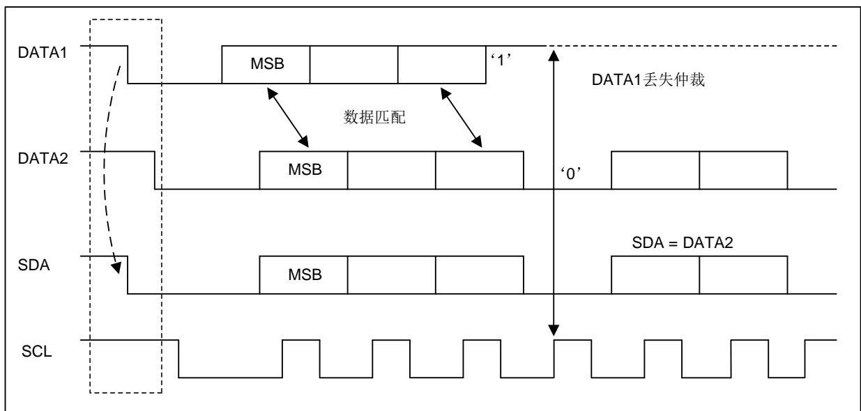
图 25-14 两个主器件仲裁
