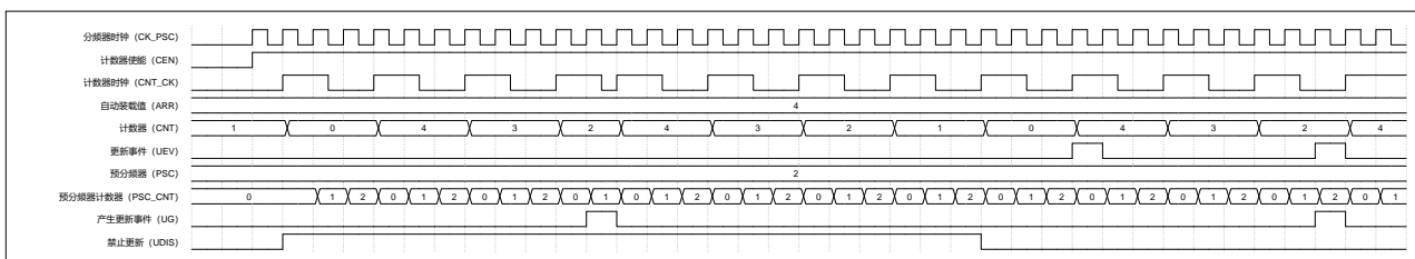
图 16-11 中央计数模式（UDIS=1 禁止产生更新事件）
