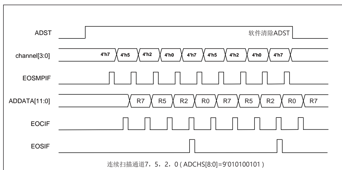
图 13-9 连续扫描模式使能通道转换时序图 (通道方向由高到低)
