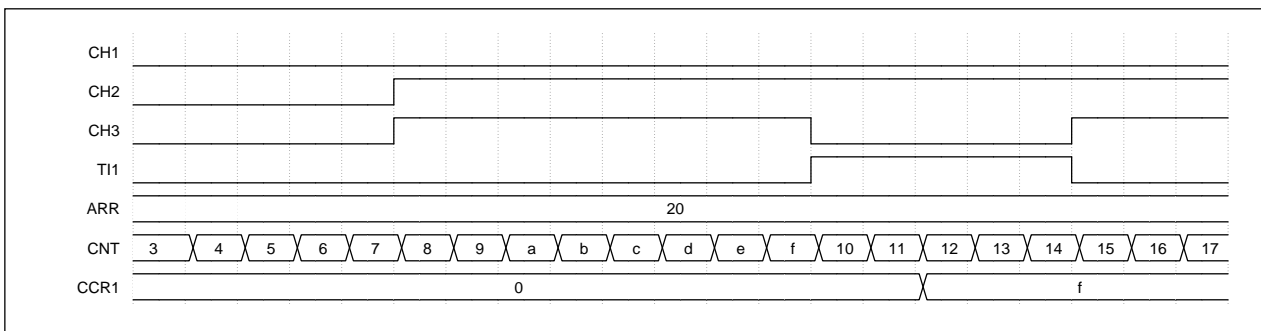
图 17-27 (TI1 异或输入) 输入捕获波形图
