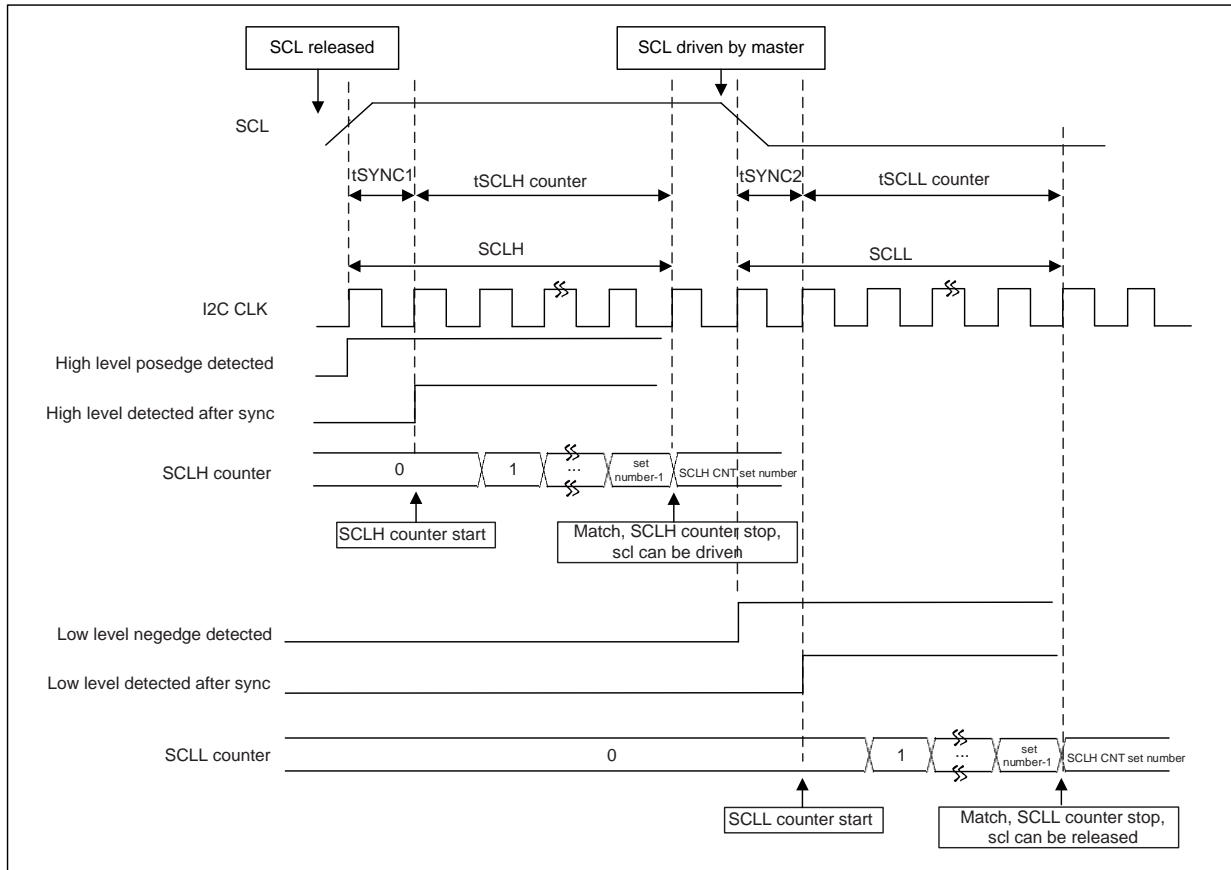
图 25-17 SCL 生成时序
