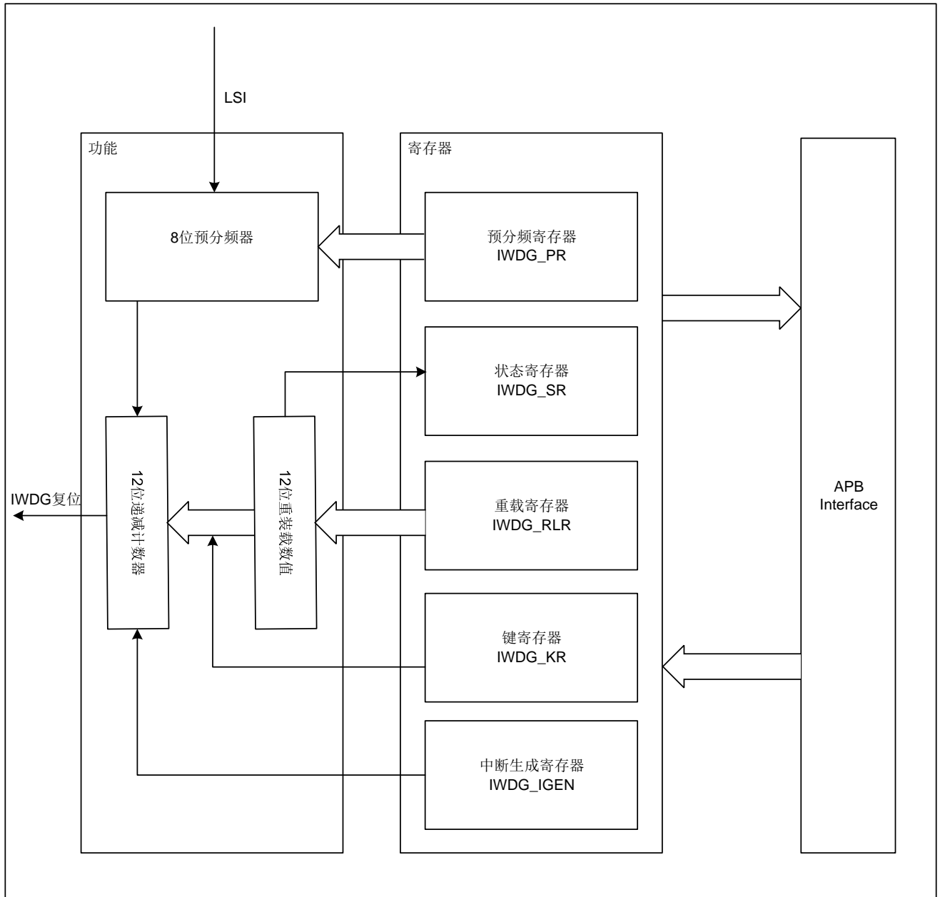
图 21-1 功能框图
