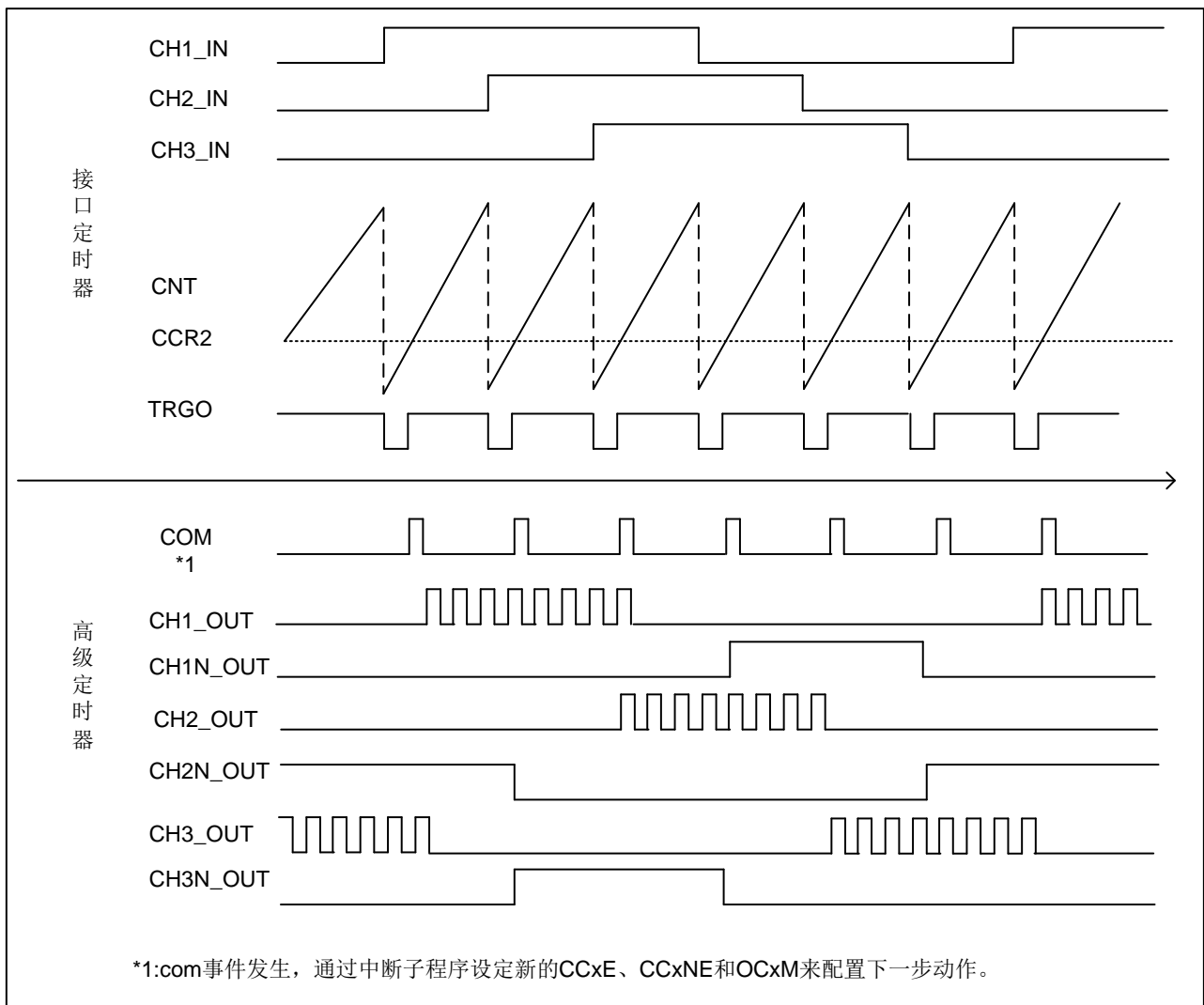
图 15-43 霍尔传感器接口实例
