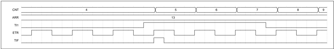
图 16-26 外部时钟模式 2+从模式（触发模式）控制时序图
