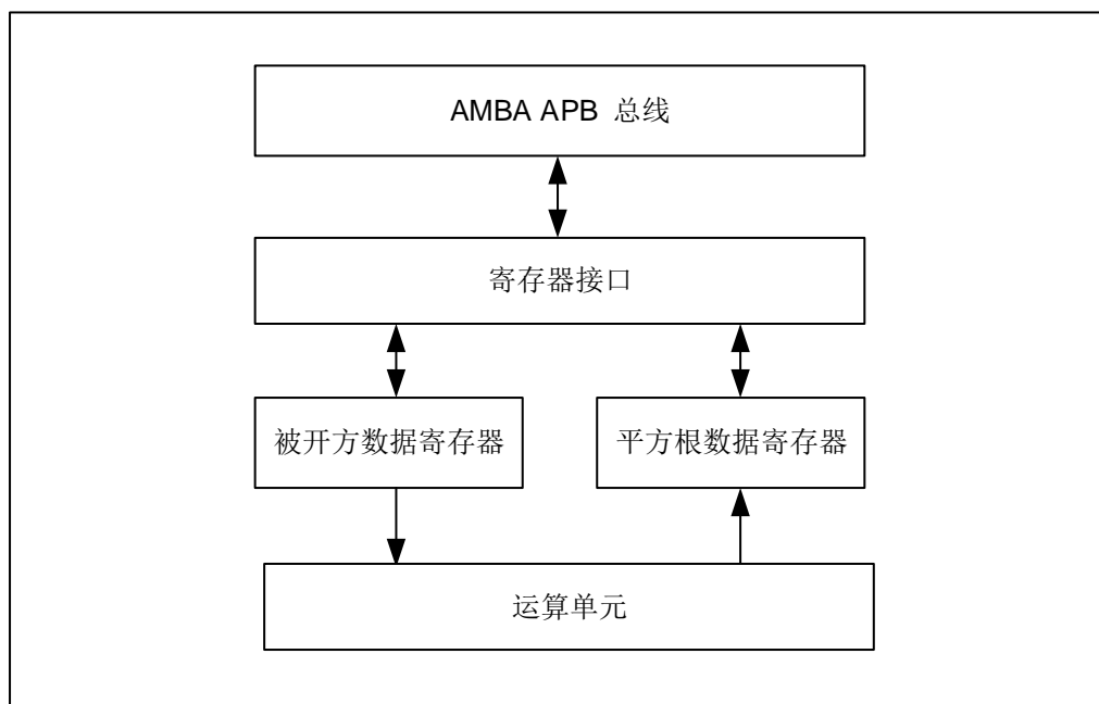
图 8-1 HWSQRT 功能框图
