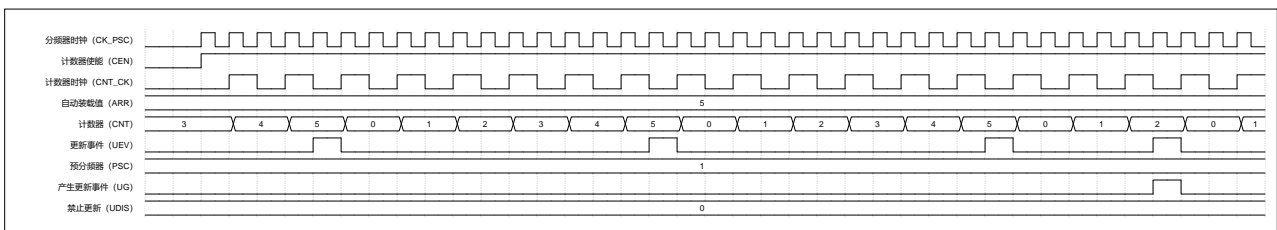
图 15-6 递增计数模式 (UDIS=0)
