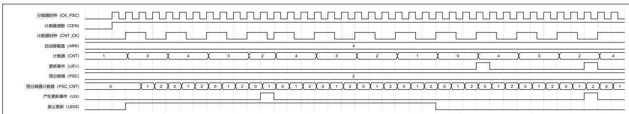
图 17-11 中央计数模式（UDIS=1 禁止产生更新事件）
