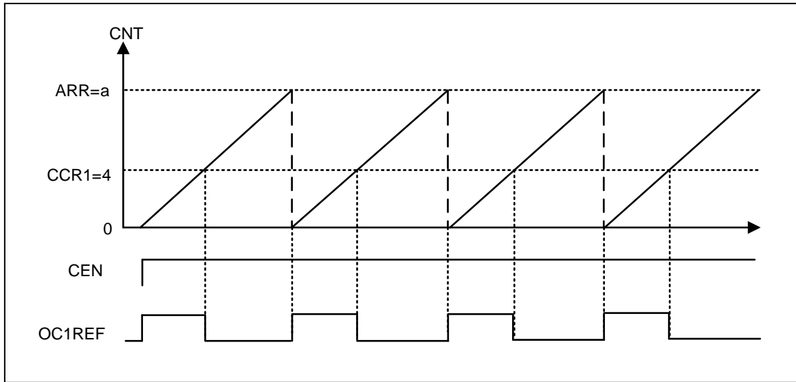
图 19-8 边沿对齐递增计数时 PWM 模式 1 的波形
