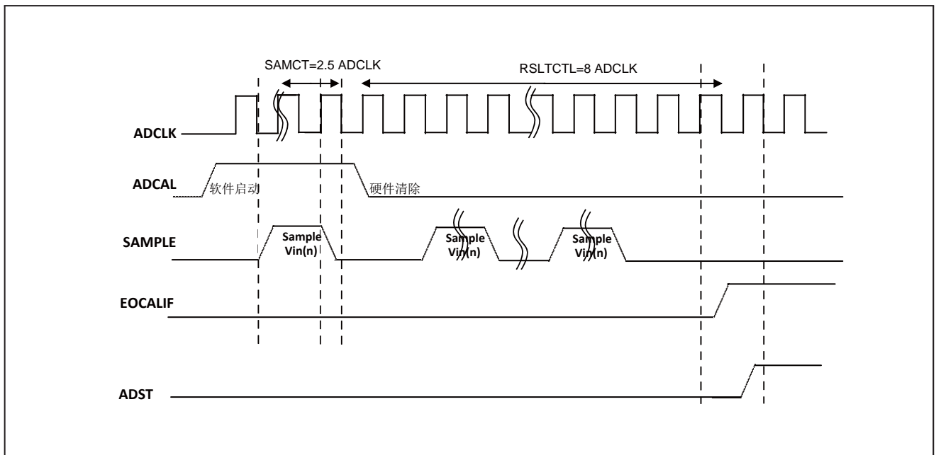
图 13-3 校准过程
