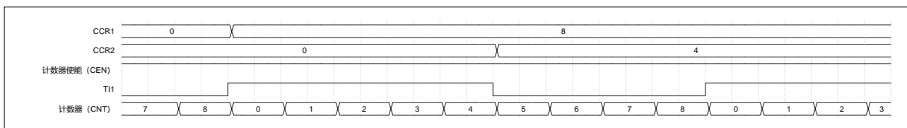
图 15-16 PWM 输入模式时序
