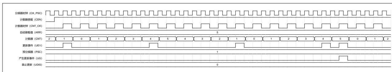
图 15-10 中央计数模式（UDIS=0）
