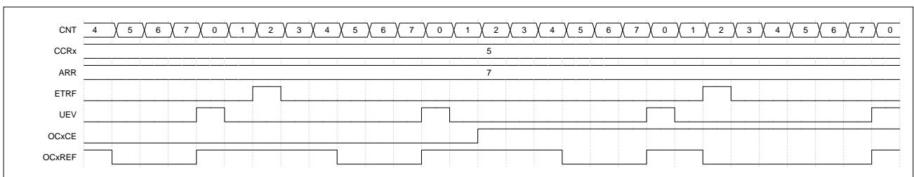
图 15-29 外部事件清除 OCxREF
