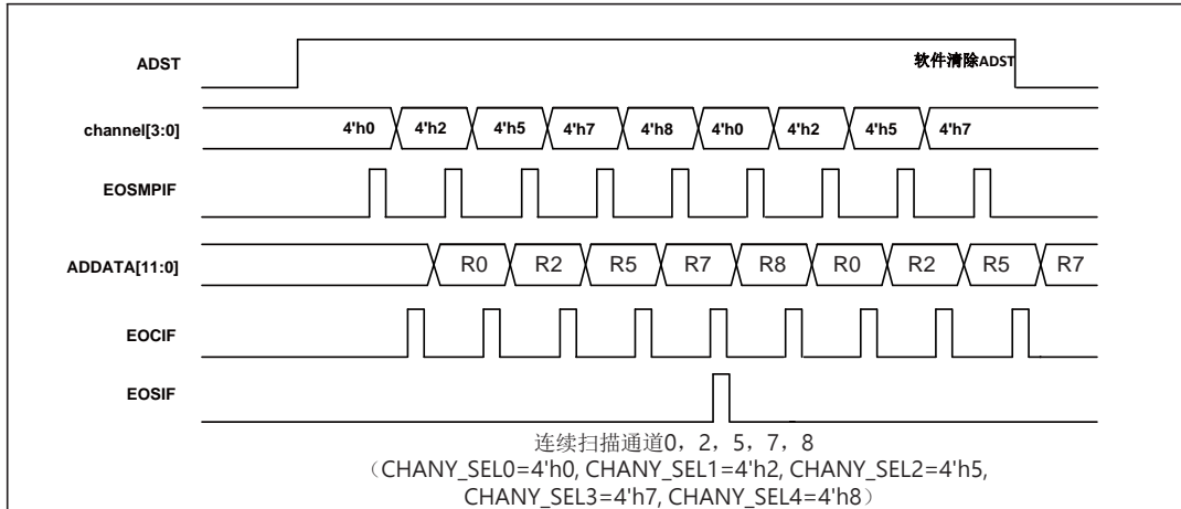
图 13-12 连续扫描模式下通道转换时序图
