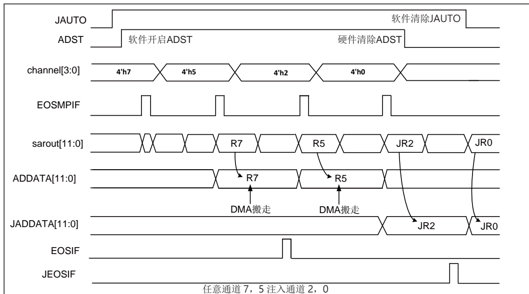
图 13-14 自动注入通道转换单周期扫描通道转换时序图
