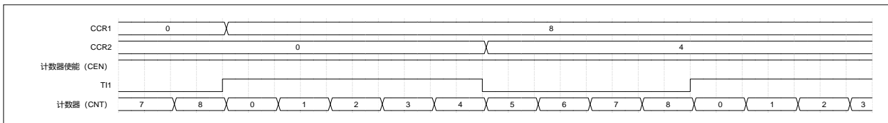
图 16-13 PWM 输入模式时序
