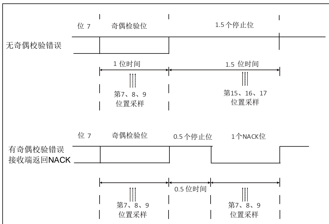
图 23-6 UART 采样 NACK 信号方框图
